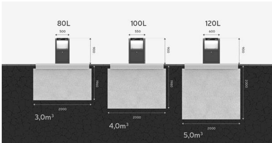
Rys. 4. Budowa pojemnika podziemnego [7]
