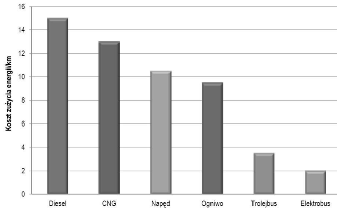
Rys.1 Koszt zużycia energii ze względu na zastosowany układ napędowy [2] Fig. 1. The cost of energy consumption due to the drive system used [2]
