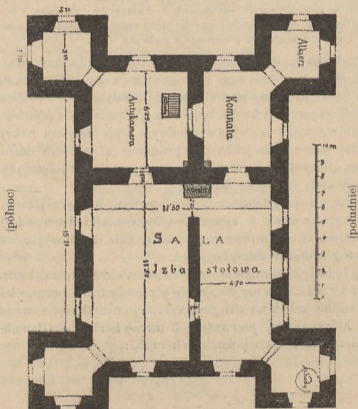
Fig. 78. Szymbark. Rzut poziomy dworu z XVI w. (str. 812) według Łuszczkiewicza.
