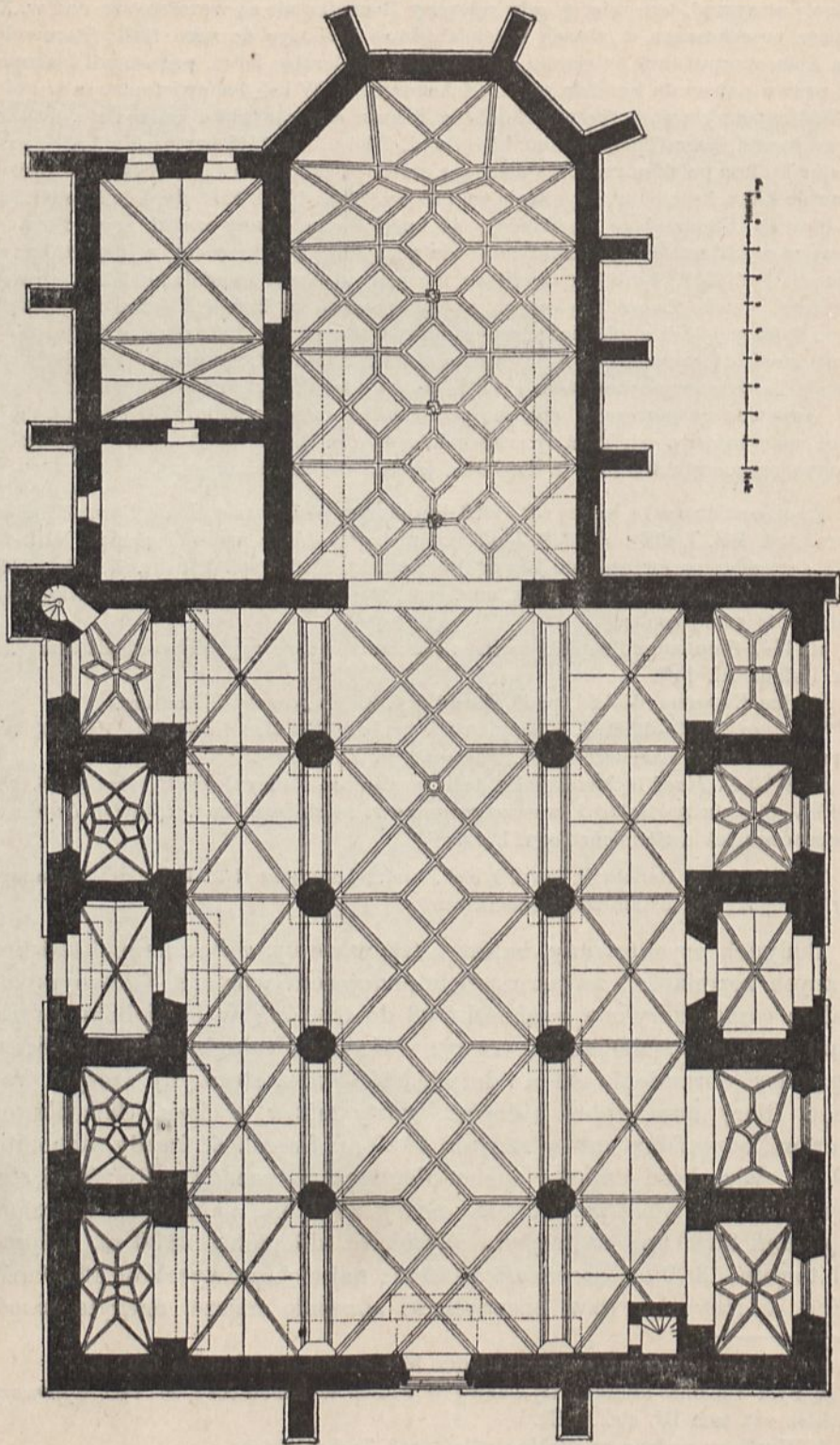
Fig. 4. Bierz. Rzut poziomy kościoła parafialnego (według Zachariewicza).
