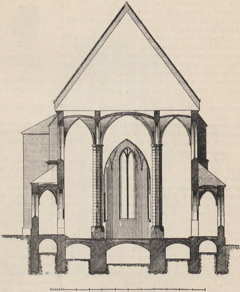
Fig. 7. Biecz. Przekrój poprzeczny kościoła parafialnego (według Łuszczkiewicza — skala: sześń wied.).
