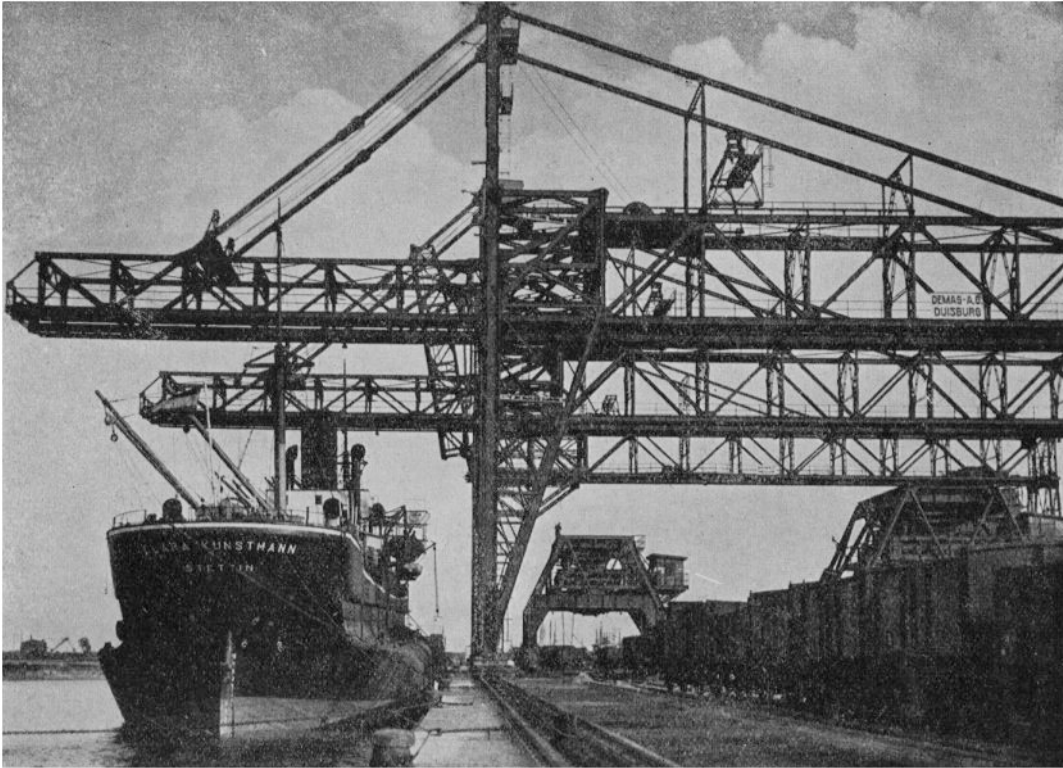
VERLADEBRÜCKEN FÜR ERZE UND PHOSPHATE
