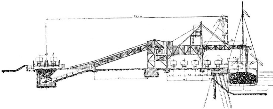
ABB. 3. — QUERSCHNITT DER NEUEN KOHLENUMSCHLAGSANLAGEN
