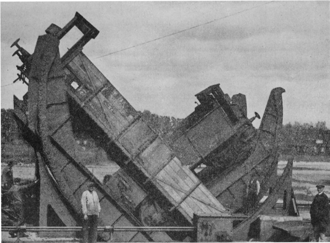
KOHLINKIPPER FÜR EISENBAHNWAGGONS
