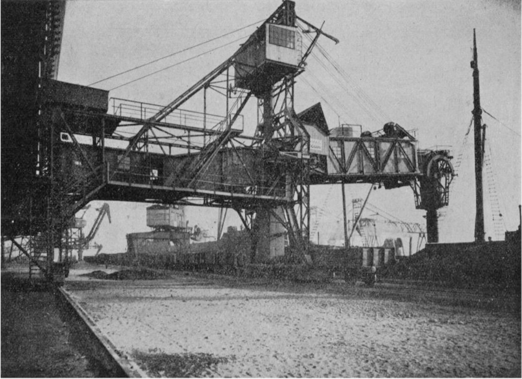
KOHLNVERLADEANLAGEN
