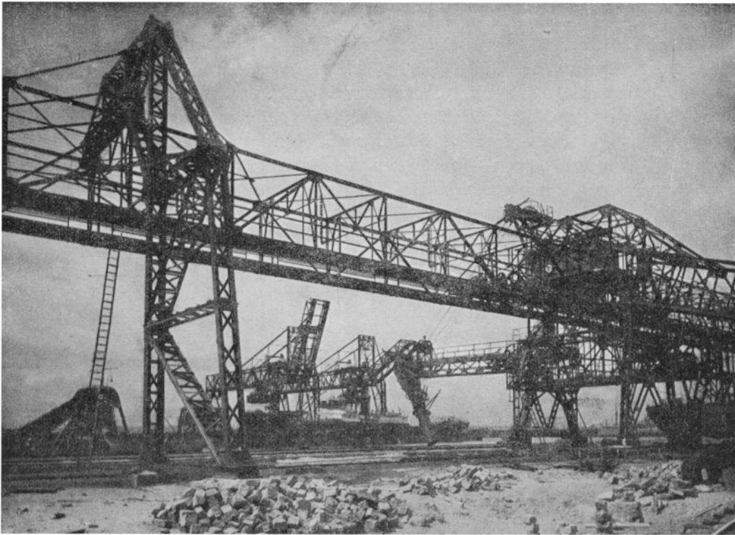
MODERNE UMSCHLAGSANLAGEN
