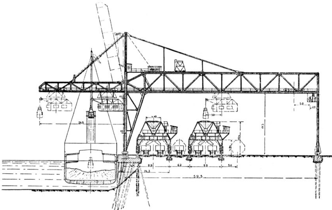
ABB. 4. — QUERSCHNITT DER NEUEN ERZVERLADEBRÜCKEN
