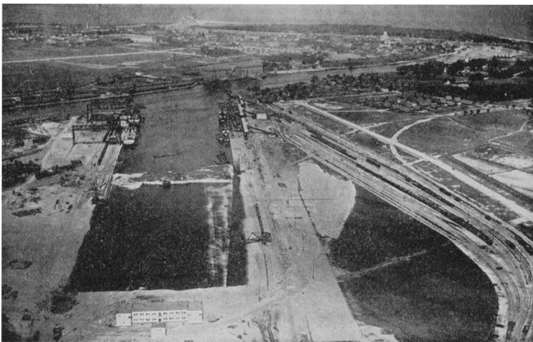
GESAMTANSICHT DES NEUEN MASSENGUTBECKENS
