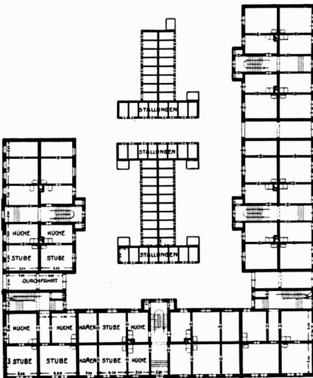
Abb. 71. Kolonie der Hubertushütte in Hohenlinde. Reihenhäuser. Grundriß.
