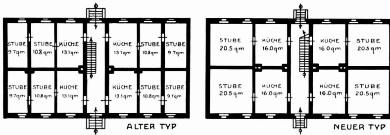
Abb. 82. Kolonie Emanuelssegen. Alte Vierfamilienhäuser vor und nach dem Umbau.
