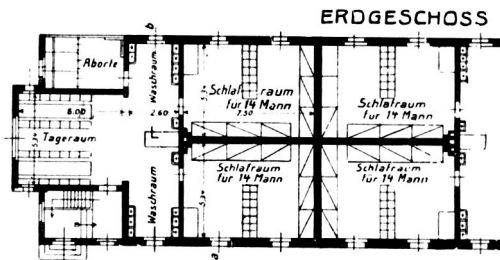
Abb. 26. Kolonie Knurów. Schlafhaus ohne Mannschaftsbeköstigung.
