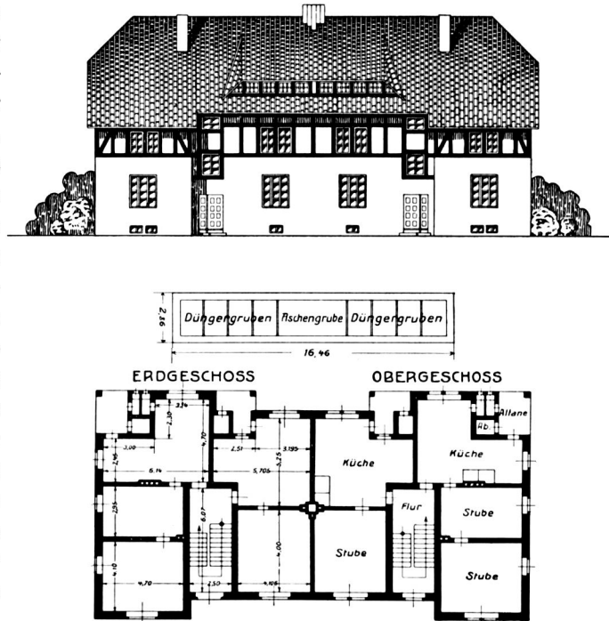
Abb. 10. Kolonie Rokittnitz. Achtfamilienhaus.
