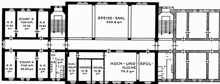
ERDGESCHOSS
