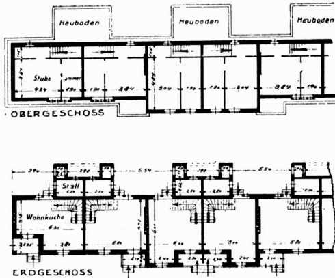
Abb. 106. Kolonie Römergrube. Grundriß zum Zehnfamilien-Reihenhaus Abb. 105.
