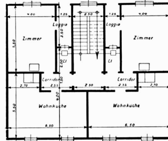
Abb. 65. Typenhaus der Hohenloherwerke A.-G. Dreistöckige Reihenhäuser in Kattowitz, Hohenlohehütte und Michalkowitz.
