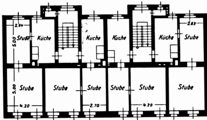
Abb. 73. Kolonie der Friedenshütte. Arbeiterwohnhaus (Reihenhaus) in Friedenshütte.
