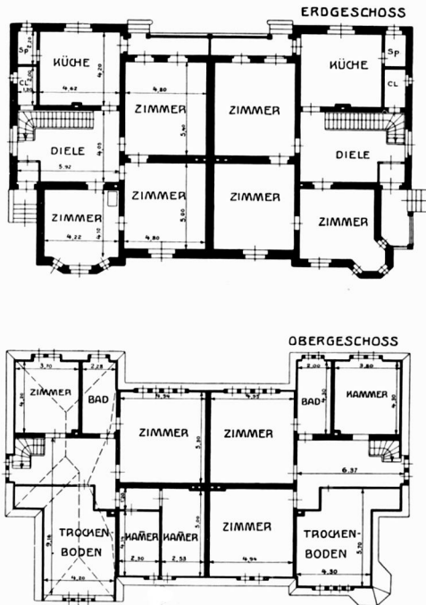
Abb. 67. Beamtenhaus der Oheimgrube. Grundriß des Hauses Abb. 61.
