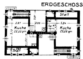
Abb. 21. Kolonie Knurów. Zweifamilienhaus. (Nr. 19 des Lageplans Abb. 14.)
