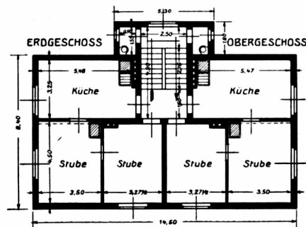
Abb. 74. Kolonie der Juliehütte. Sechsfamilienhaus.
