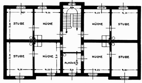
Abb. 70. Kolonie Carlssegen. Achtfamilienhaus.
