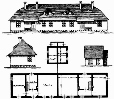
Abb. 46. Gieschewald. Zweifamilienhaus.
