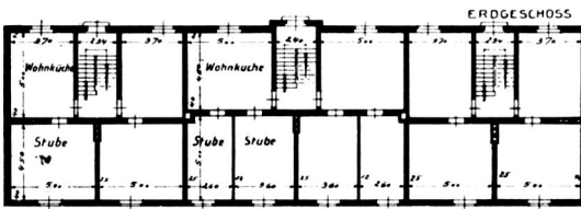
Abb. 99. Kolonie Emmagrube. Zwölffamilienhaus (Dreihäusertyp).
