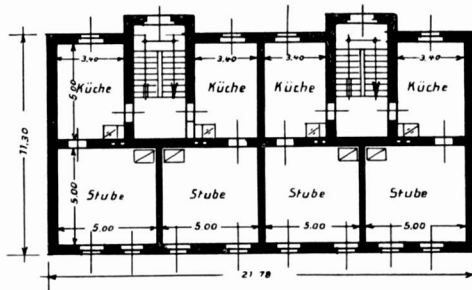
Abb. 120. Kolonie der Dubenskogrube. Achtefamilienhaus.
