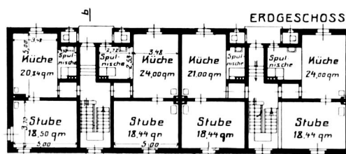
Abb. 24. Kolonie Knurow.
