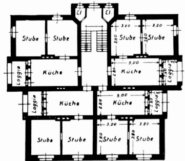
Abb. 34. Kolonie der Donnersmarckhütte. Zwölffamilienhaus. Typischer Grundriß,
