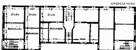
Abb. 111. Kolonie Annagrube. Zwölffamilienhaus (Dreihäusertyp).
