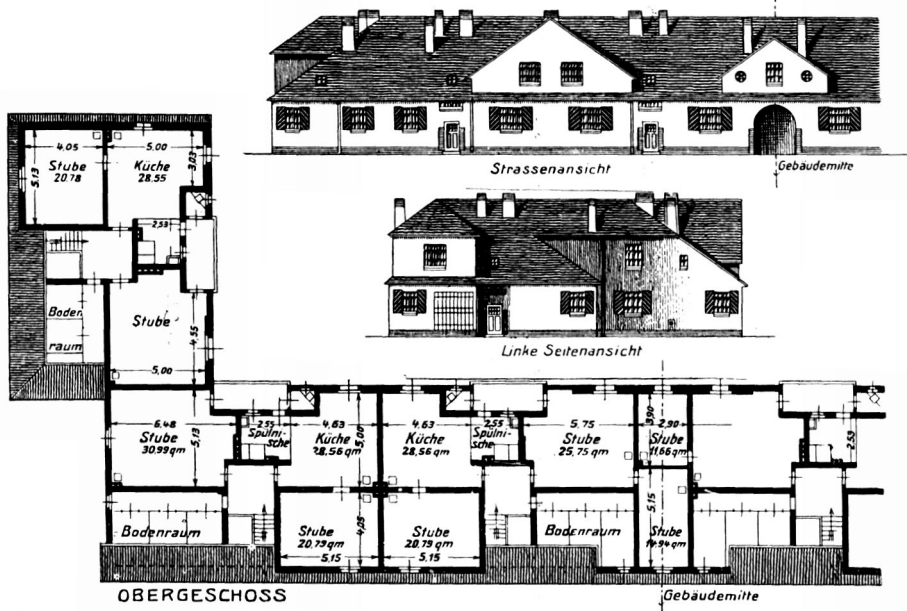
Abb. 25. Kolonie Knurow. Achtehnfamilienhaus. (Nr. 30 des Lageplans.)
