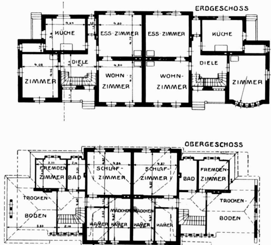
Abb. 68. Beamtenhaus der Oheimgrube. Grundriß des Hauses Abb. 59.
