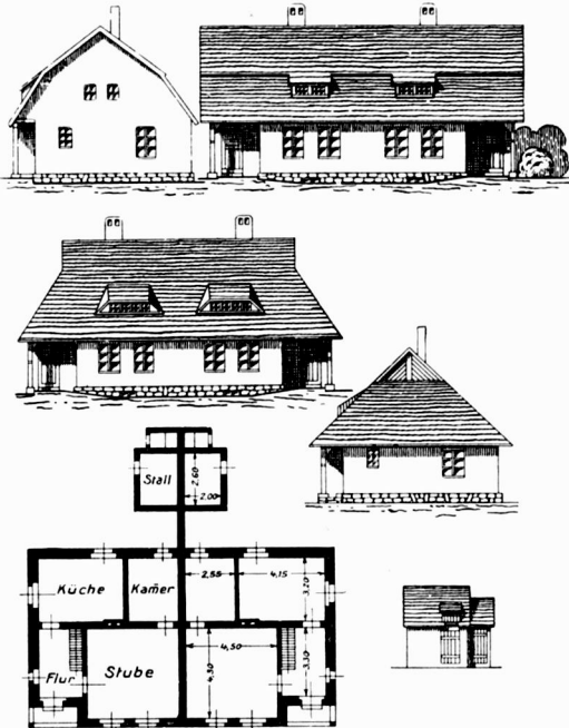
Abb. 47. Gieschewald. Zweifamilienhäuser.
