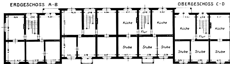
Abb. 13. Bialas-Kolonie. Zwanzigfamilienhaus.
