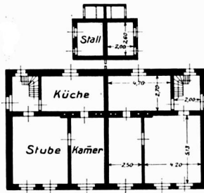
Abb. 48. Gieschewald. Zweifamilienhäuser.
