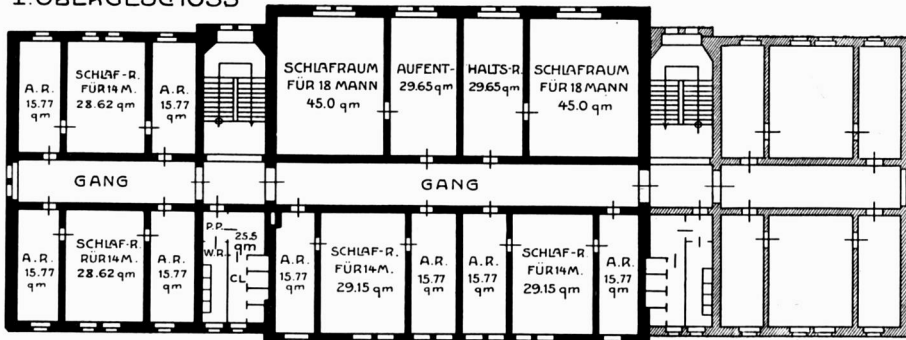
Abb. 90. Kolonie Kostuchna. Schlafhaus mit Mannschaftsbeköstigung.
