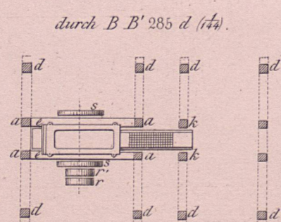
durch B B' 285 d (1/4)
