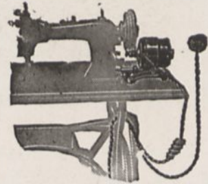
Universal-D. R. G. M. - Näh- maschinenmotor m. Kugel- lagerung, Fussregler usw. Ohne Montage sof. betriebsbereit. Für angestrengten gewerblichen Dauerbetrieb; verbraucht in etwa 66 Betriebsstunden nur 1 Kw-Std. annähernd 1/12 P. S. - Leistung Man verlange Anerkennungs- schreiben!
