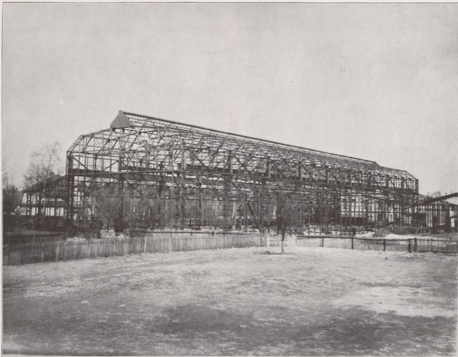
Bild 2 Montagehalle II — Zawadzki
