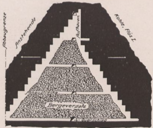
Abbau im Flöz selbst. Fig. 4. (folgt der Ebene von Flöz I).
