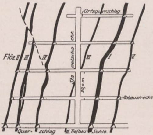
Fig. 3. Stapelschicht (Saigerriss)
