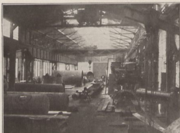
Teilansicht: Abt. Kesselschmiede
