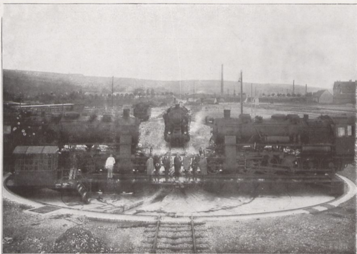
Bild 3 Lokomotiv-Drehlscheibe, 23 m Durchmesser, 240 t Tragkraft
