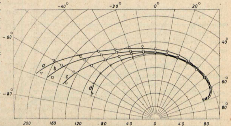
Rys. 3. Jasność (wyrażona w % od wartości odpowiadającej \varphi = 55^\circ ) szkła mlecznego różnie matowanego w zależności od \varphi dla \Psi = 0^\circ i \Theta = 55^\circ ; a) matowanie przez firmę F. Schmidt i Haensch; b) matowanie przy pomocy karborundu (wymiar liniowy ziaren około 0,1 mm); c) matowanie strumieniem piasku; d) matowanie chemiczne.
