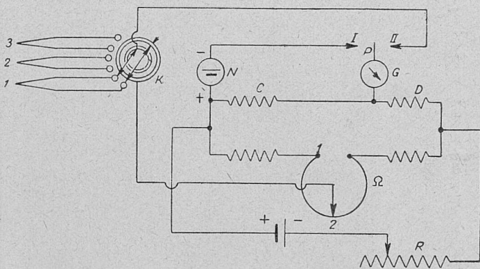
Rys. 11. Schemat potencjometru.
