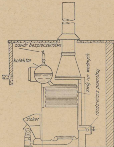
Kocioł Lamont
