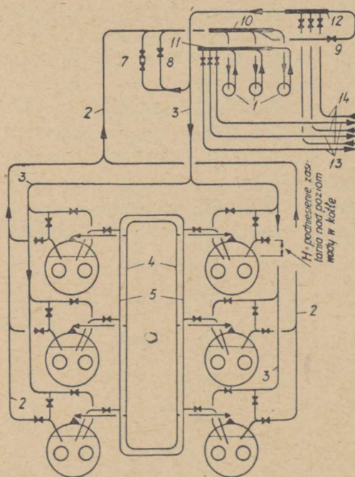
Schemat urządzenia kotłowni - kotły Super-Economia 1-Pompy cyrkulacyjne 2-Zasilenie 3-Powrót 4-Rura wyrównawcza parowa 5-Rura wyrównawcza wodna 6-Termoseparat na mieszaniu obiegiu głównego wody 7-Obejście zapasowe ręcznie obsługiwane 8-Połączenie pomocnicze zabezpieczające doprowadzenie wody powrotnej do zasilania 9-Rozdzielacz na ssaniu pomp 10-Rozdzielacz na tłoczeniu pomp 11-Rozdzielacz powrotny 12-Zasilenie 13-Powrót
