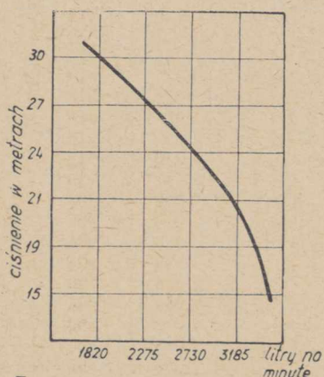
Typowa krzywa charakterystyczna pompy cyrkulacyjnej.
