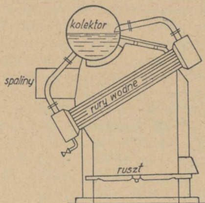
Kocioł wodno-rurkowy Fraser.
