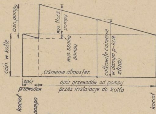
Rozkład ciśnienia pompy.
