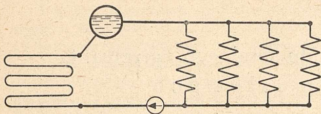
Rys. 3. Schemat kotła La Mont
