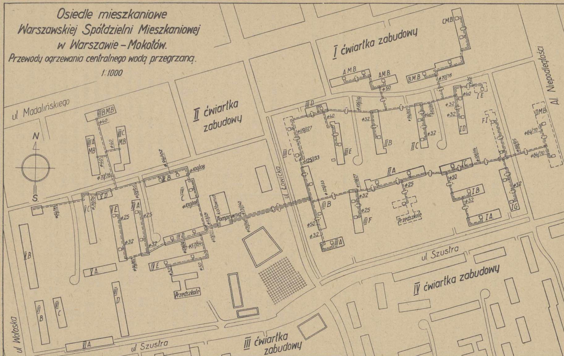
Przewody ogrzewania zdalaczynnego Osiedla Mieszkaniowego Warszawskiej Spółdzielni Mieszkaniowej (Warszawa—Mokotów)
