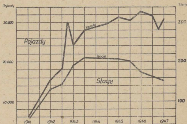
Ilość stacji kompresorów Ilość pojazdów poruszanych gazem sprężonym.
