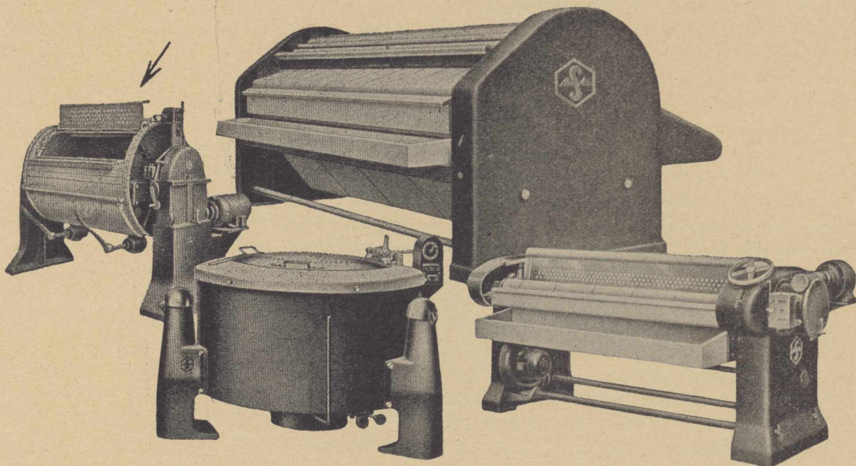
Rys. 11. Gazowa maszyna pralnicza z centryfugą, gorącym magłem i prasą uniwersalną.
