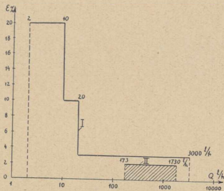
Rys. 1. Zależność dopuszczalnego błędu od natężenia przepływu: I według przepisów paryskich, II według przepisów G. U. M.
