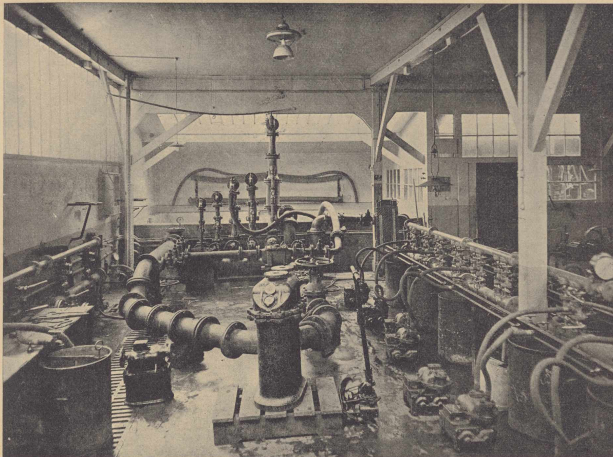
Rys. 2. Pracownia dla sprawdzania wodomierzy Zakładu wodociągowego m. Paryża.
