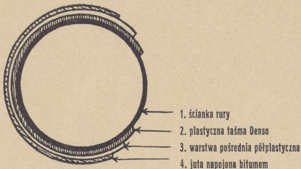
Rys. 1. Kombinowana powłoka ochronna „Denso”.
