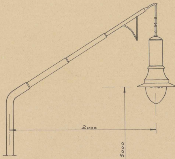
Rys. 7. Słup latarni z wysięgiem.
