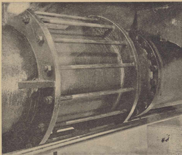
Rys. 3. Zesuwka kołnierzowa zamontowana na stacji pomp Zakładu Wodociągowego m. Lwowa.
