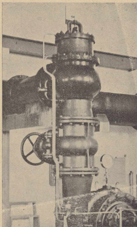
Rys. 2. Zwrotny zawór kątowny wmontowany na stacji pomp Zakładu Wodociągowego m. Lwowa.
