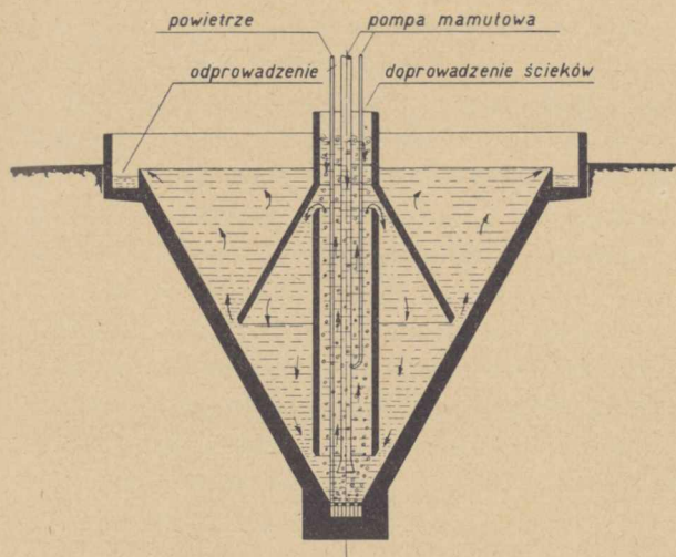
Rys. 3. Osadnik wtórny.
