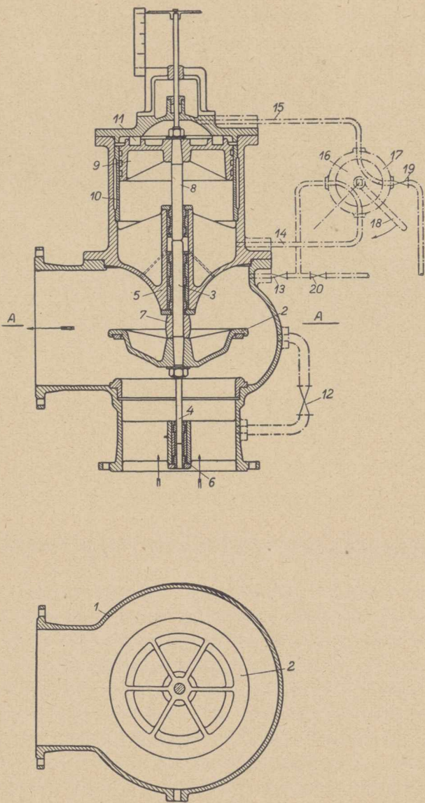
Rys. 1. Zwrotny zawór kątowny w przekrojach.
