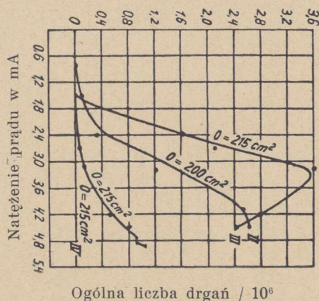
Rys. 2. I — taśmy przepojone bitumem Shirting (4 mm). II — bitum podwójny (2,5 mm). III — juta przepojona bitumem (4 mm). IV — kombinowana powłoka ochronna „Denso” (4 mm).
