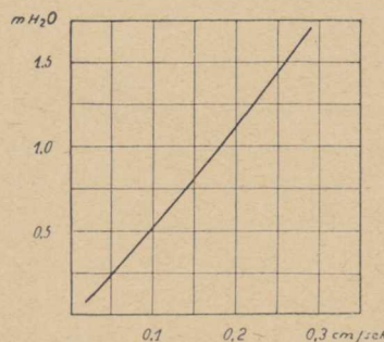
Rys. 5. Krzywa spiętrzenia w zależności od liniowej prędkości przepływu wody, przy 50 cm warstwie węgla BSW 061.
