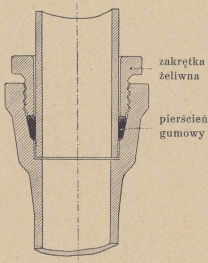
Rys. 1. Kielich typu „Union”.
