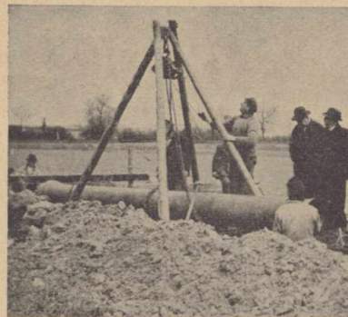
Rys. 7. Układanie przewodu z rur żeliwnych \varnothing 400 mm z elastycznymi połączeniami „Union” w Hamm.
