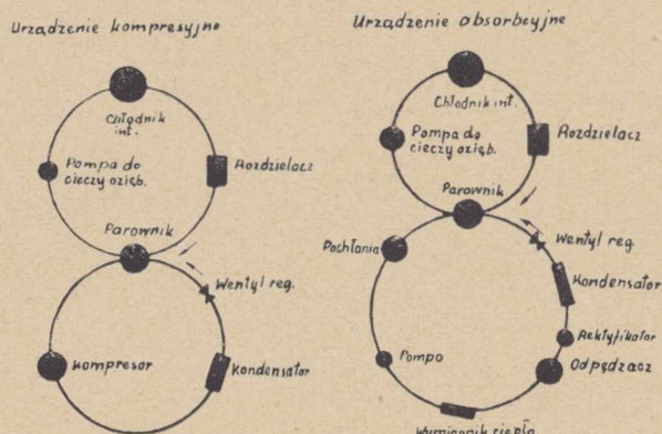
Rys. 1. Schemat obiegu amoniaku (dolne koła) i cieczy oziębiającej (górne koła)
