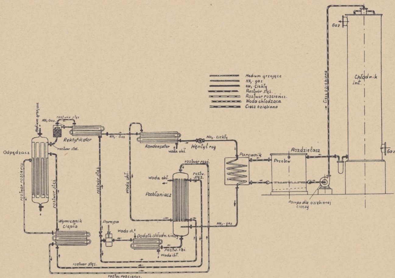
Rys. 2. Schemat urządzenia chłodniczego syst. Dra Lenza.
