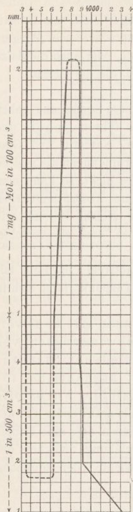
Fig. 50. Morphin.
