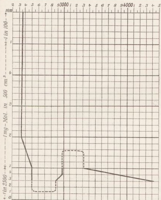
Fig. 68. Corydinsäure.
