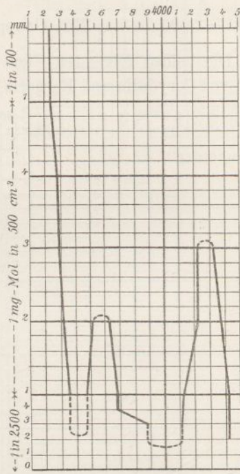
Fig. 71. Veratrinsäure.
