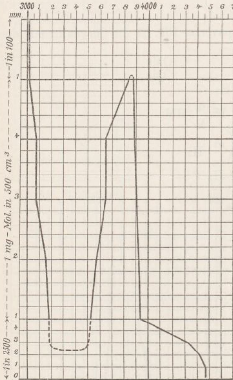
Fig. 60. Hydrastin.
