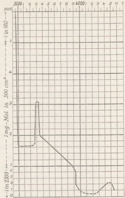
Fig. 55. Papaverin.
