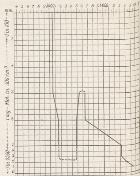
Fig. 65. Oxyhydrastinin.
