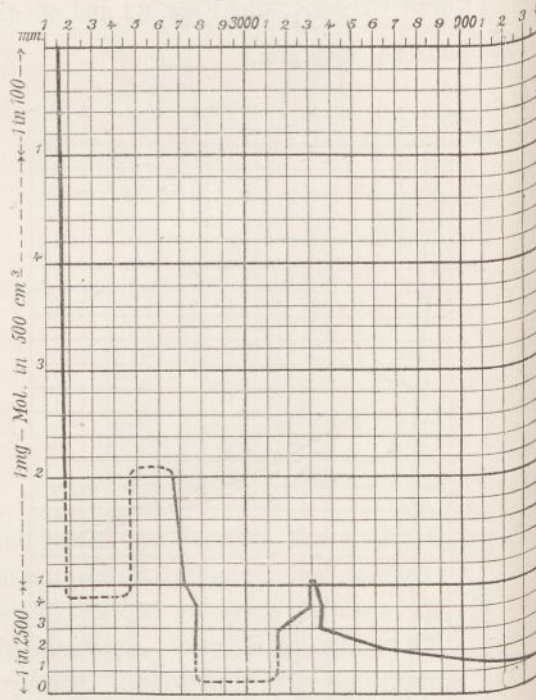
Fig. 67. Berberin nitrat.
