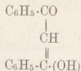
\alpha -Oxybenzalacetophenon, Schm. P. 77—78° enolisch
