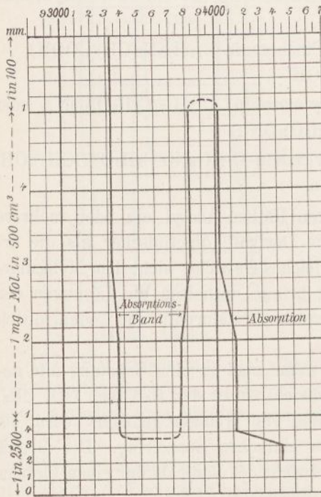
Fig. 56. Tetrahydropapaverin.
