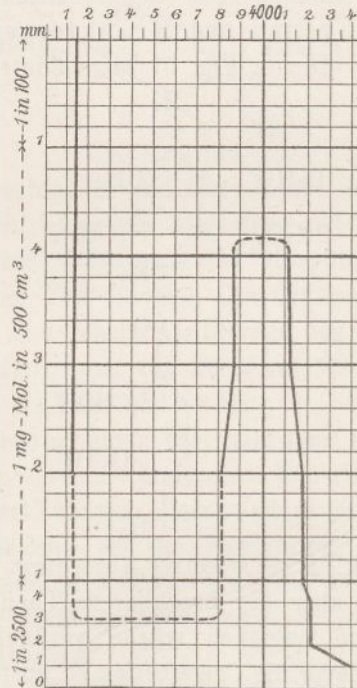
Fig. 53. Cinchonin.
