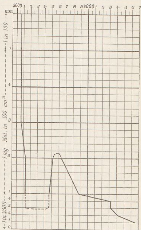
Fig. 63. \omega -Aminoäthylpiperonylcarboxylanhydrid.
