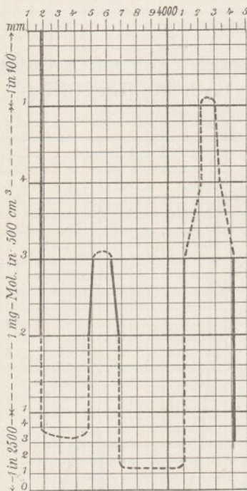
Fig. 70. Piperonylsäure.
