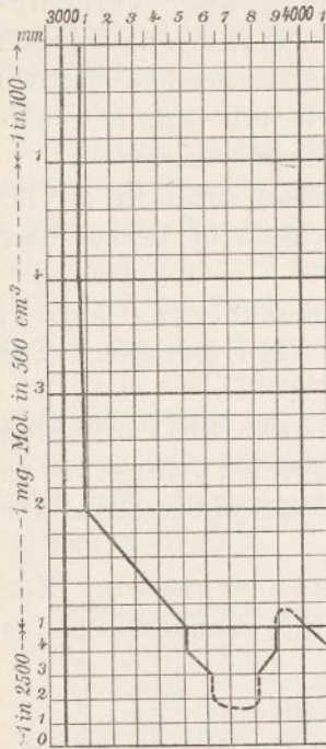
Fig. 54. Bulbocapnin.
