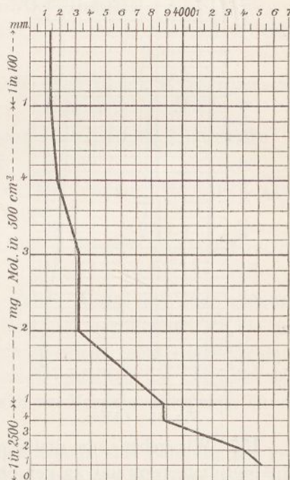
Fig. 51. Narceïn.
