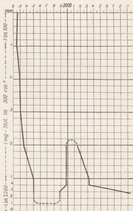
Fig. 69. Berberidinsäure.
