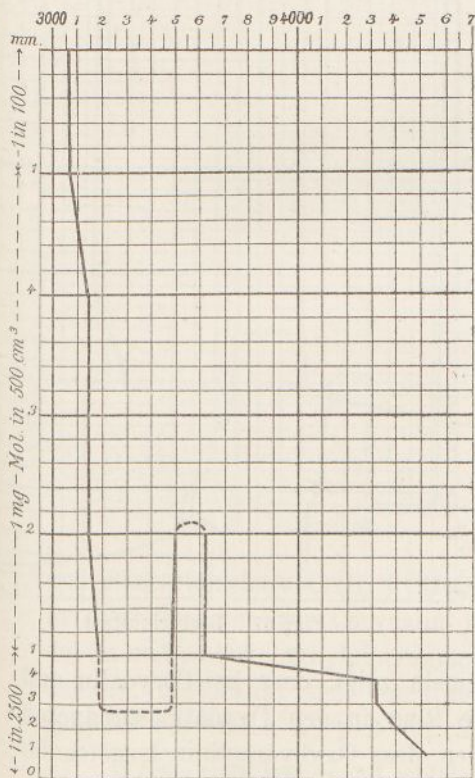
Fig. 62. Corydaldin.
