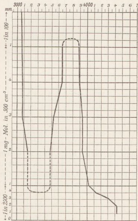
Fig. 59. Narcotin.
