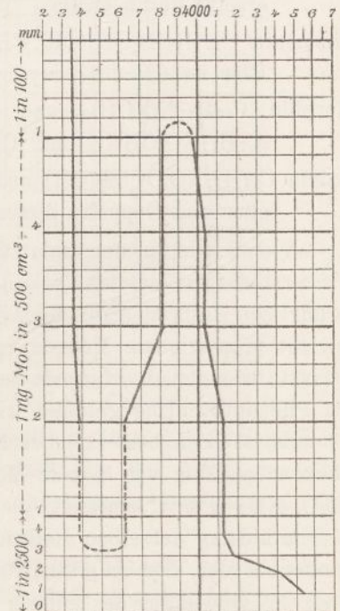
Fig. 57. Corydalin.
