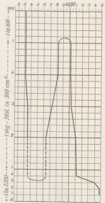
Fig. 61. Corybulbin.
