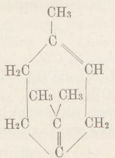
\Delta^{1.4} (8)-Terpadien
