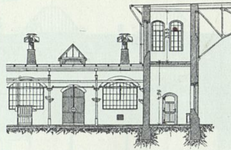
Teil des Längenschnittes durch den Auschlachte-raum.
