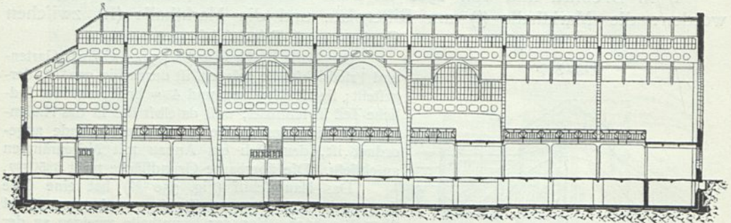
Längenschnitt.
