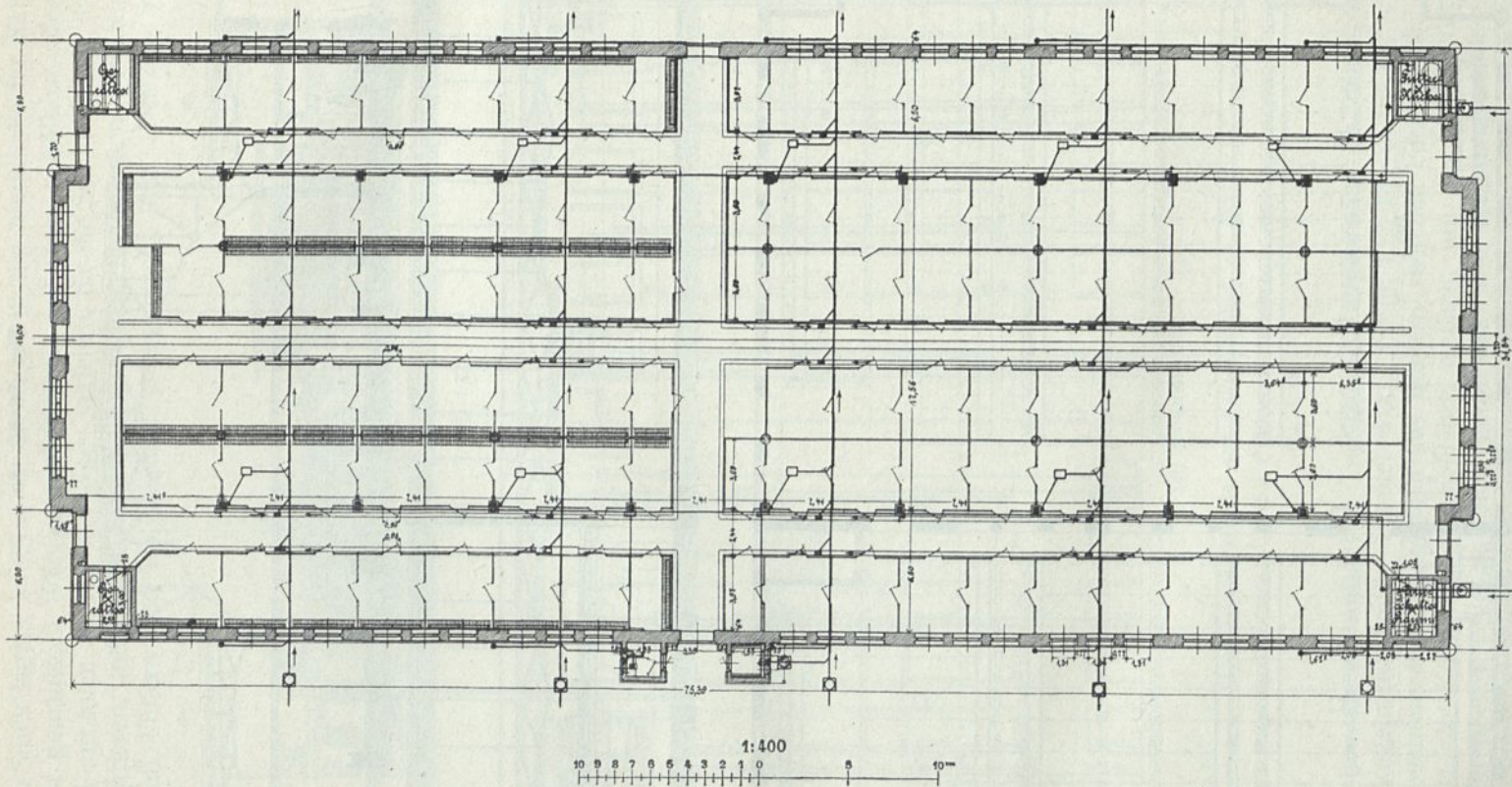
Kleinvieh-Markthalle auf dem Viehhof zu Breslau 11).
