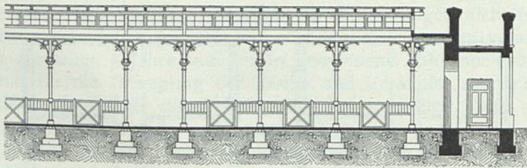
Teil des Längenschnittes.
