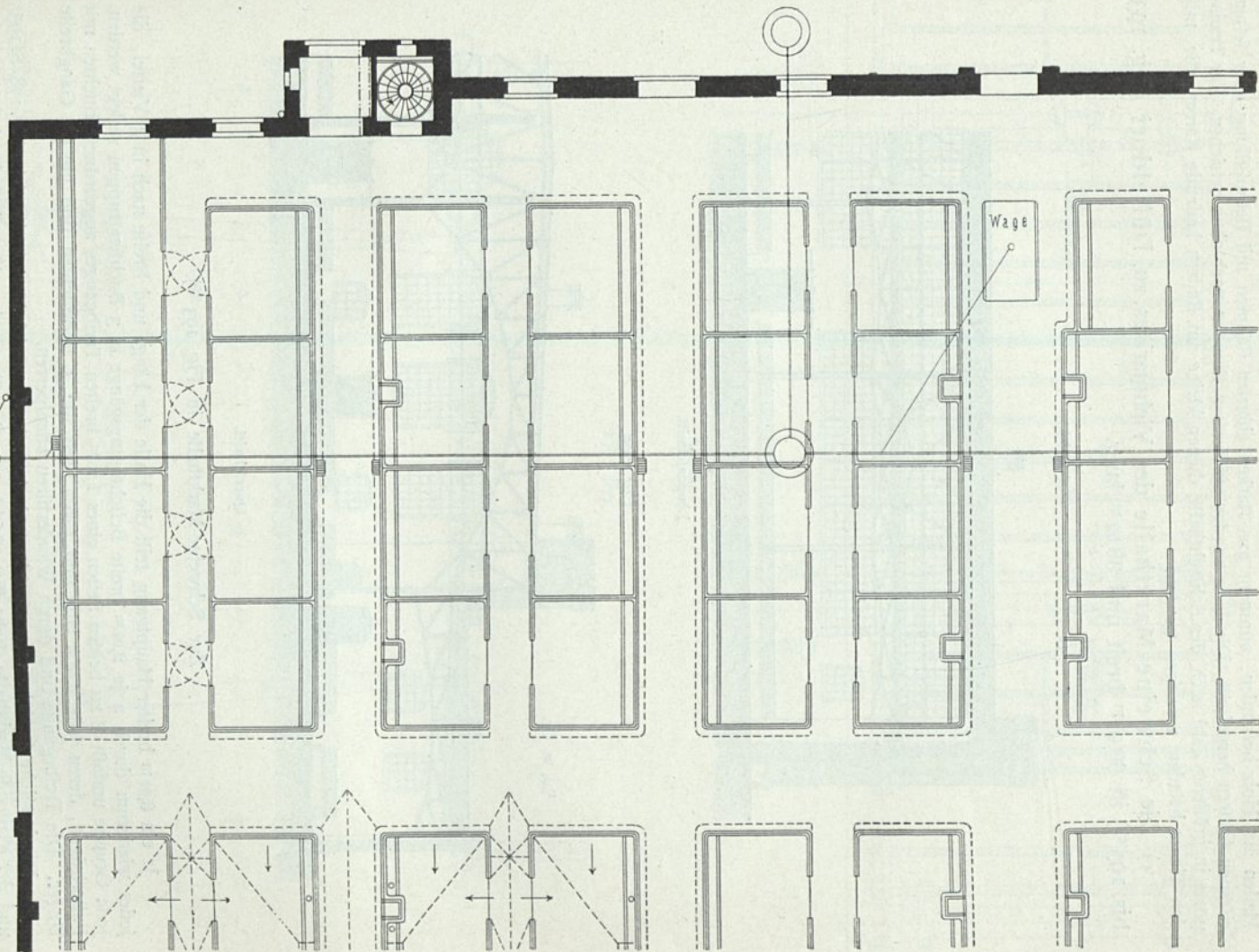
Viertel des Grundriffes der Schweine-Markthalle auf dem Viehhof zu Düffeldorf 34) .
