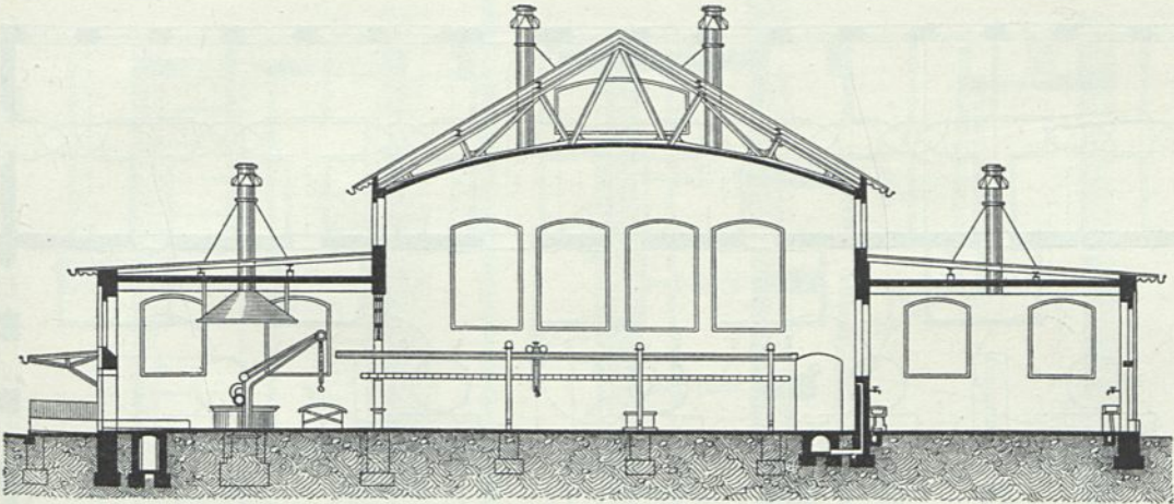
Querschnitt.
