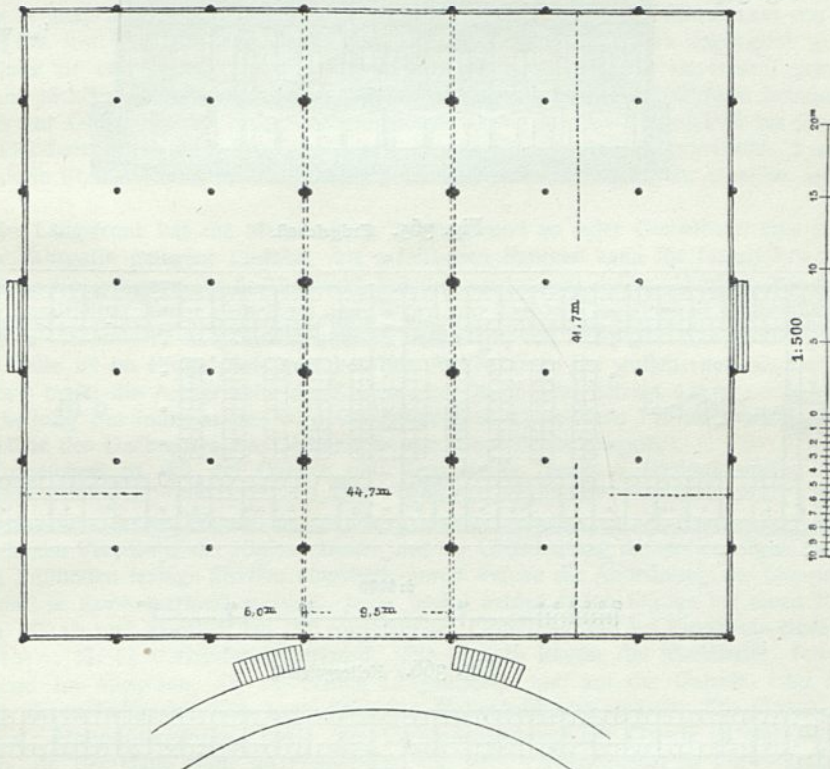
Markthalle zu Stuttgart 248 ).
