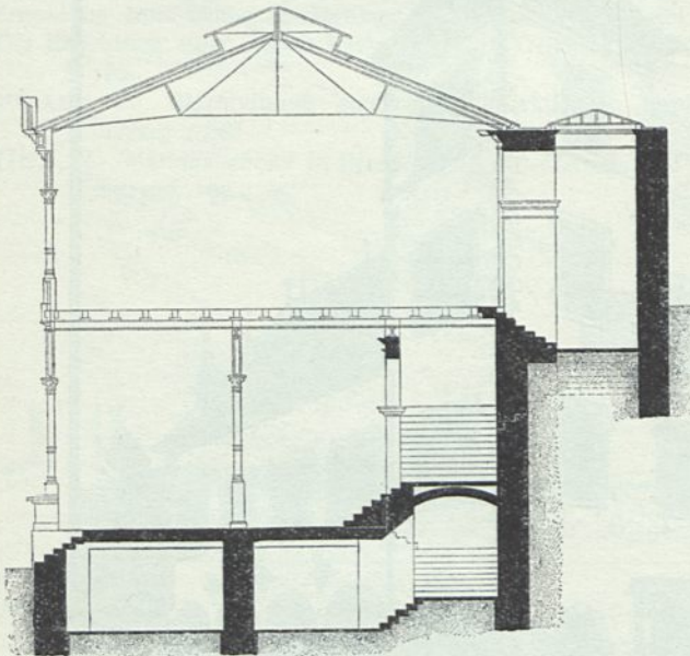
Fig. 361. Querschnitt.
