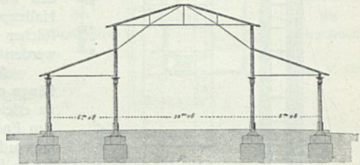
Querschnitt zu Fig. 381 u. 382.
