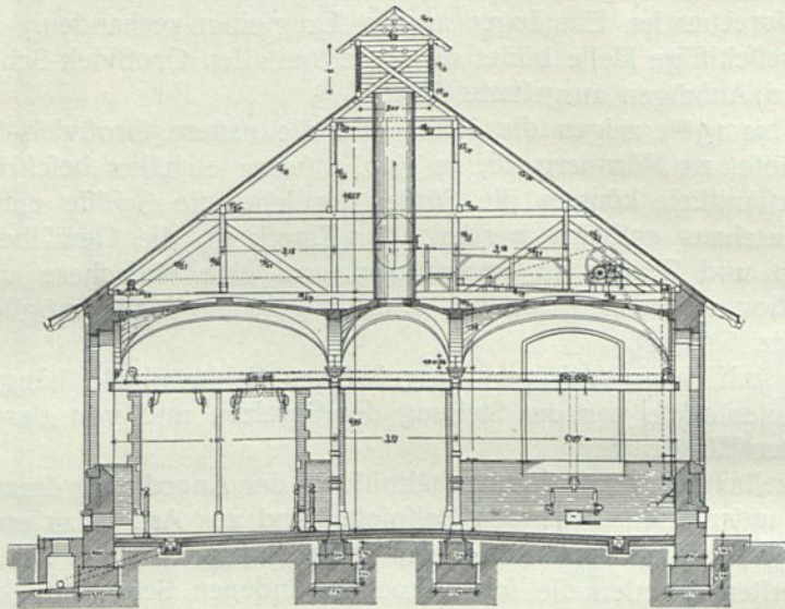
Querschnitt.
