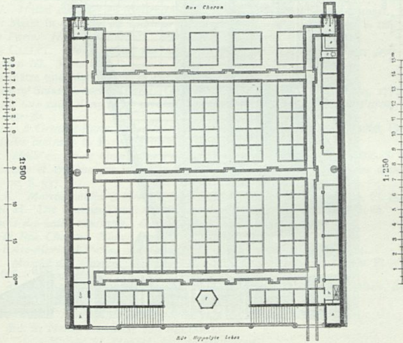
Markthalle des Martyrs zu Paris 108) .
