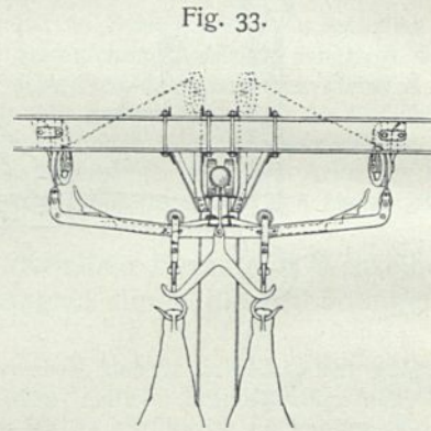
Abgabe der Tierhälften von der Spreize an die Laufkatze.
