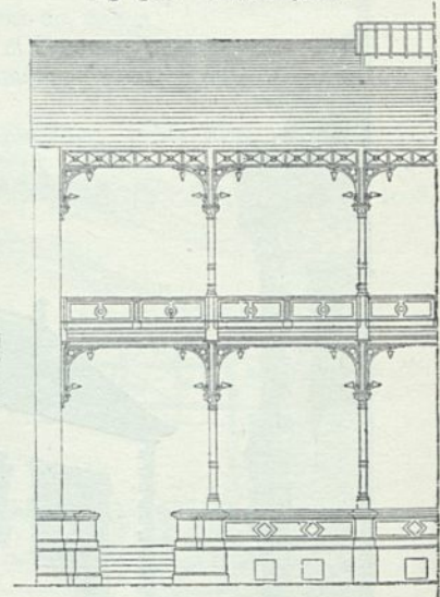
Fig. 362. Faffungsystem.
