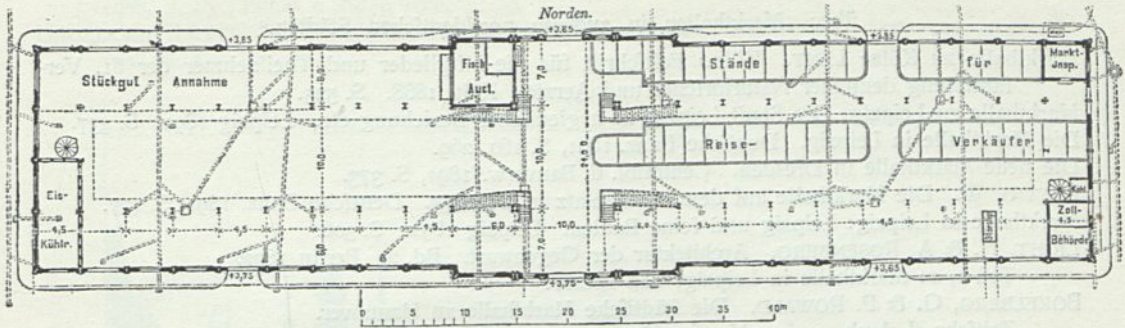
Markt- und Versteigerungshalle für Fische zu Altona 242) .
