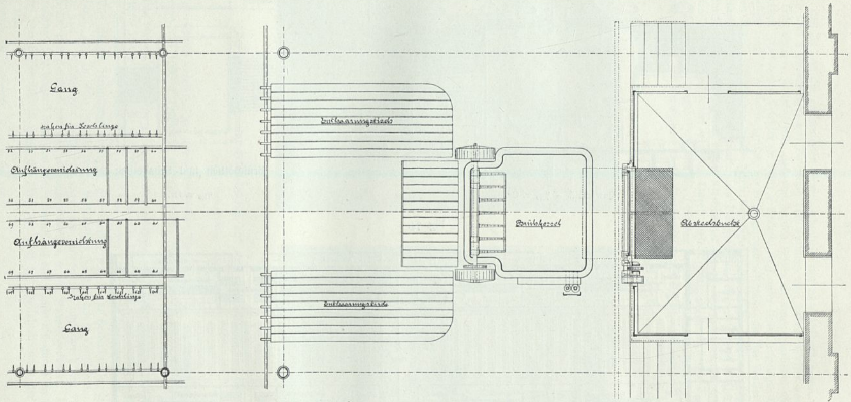
Grundriß.
