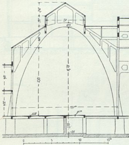
Hauptbinder der Markthalle II zu Breslau 238) .
