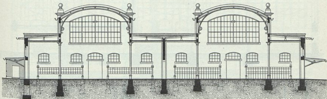
Querschnitt der Kleinvieh-Markthalle auf dem Viehhof zu Plauen 42) .
