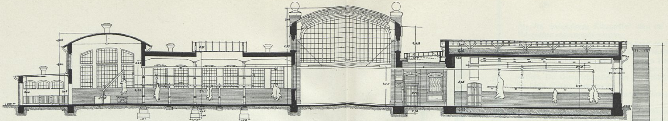
• SCHNITT A-B •
