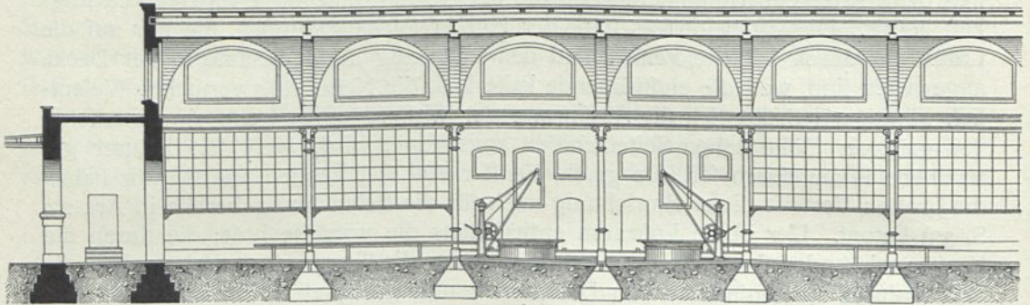
Längenschnitt.
