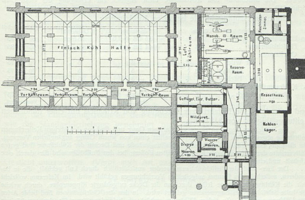
Kühlanlage in der städtischen Großmarkthalle zu Wien 165) .
