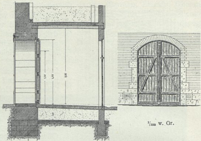
Kühlhauseingang im Schlachthof zu Breslau 11) .
