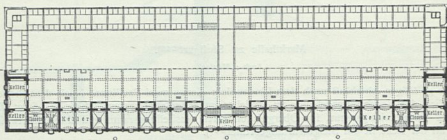
Fig. 366. Kellergeschoß.
