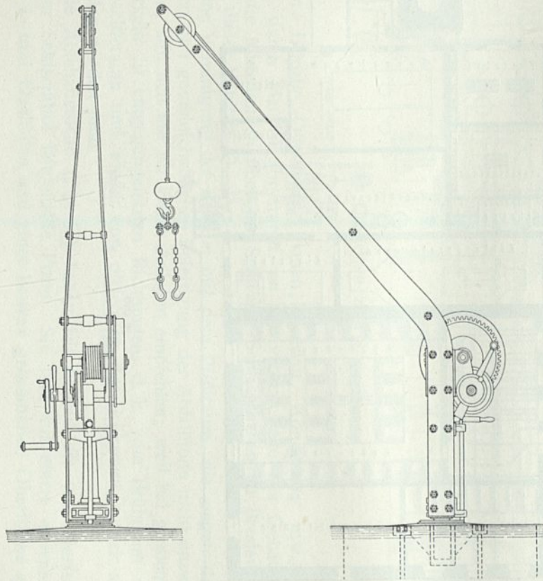
Freiftehender Drehkran
