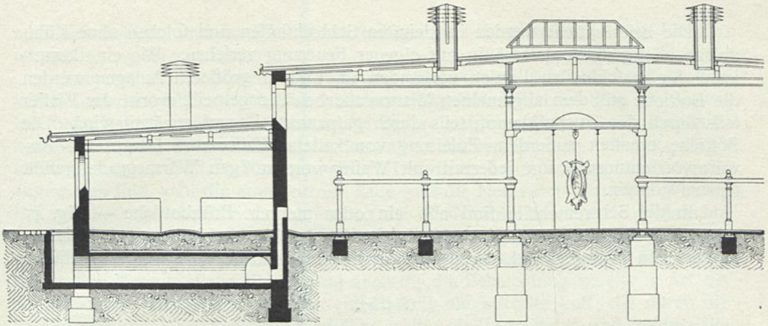
Querschnitt.
