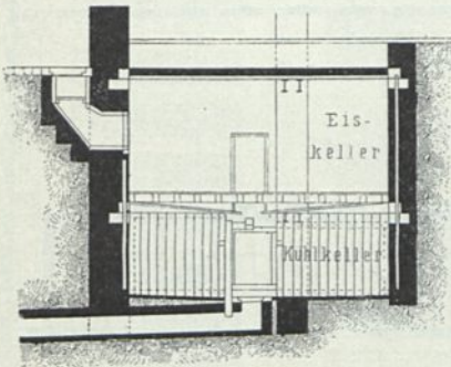
Fig. 318. Schnitt durch die Eiskeller.
