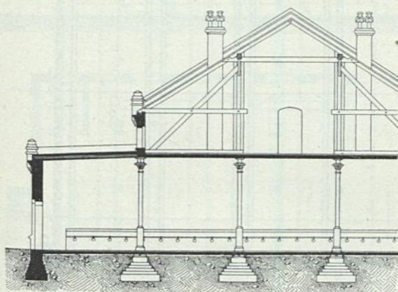
Querschnitt.
