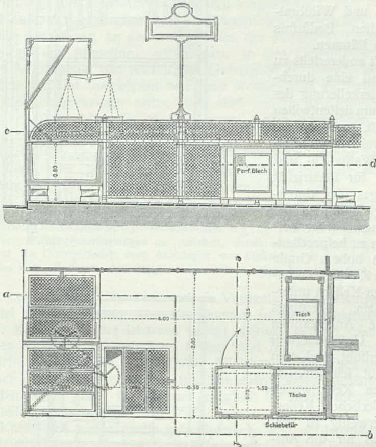
Fleischverkaufsstand in der neuen Hauptmarkthalle zu Cöln 1883).
