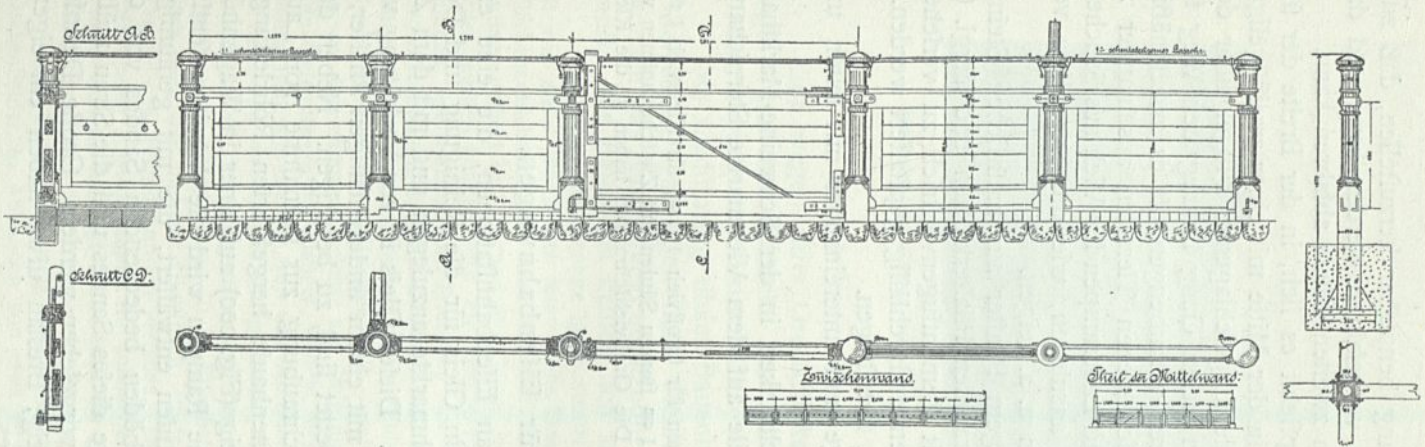
Konstruktion der Kälberhürden auf dem Viehhof Sternfchanze (Hamburg 87).
