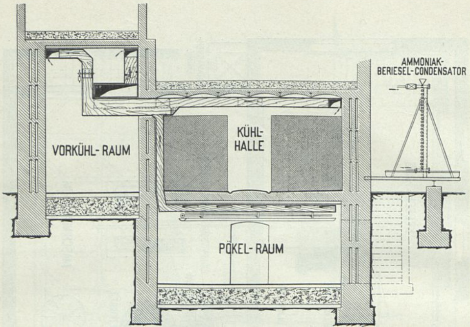
Querschnitt durch die Kühlräume in Fig. 91 u. 92.
