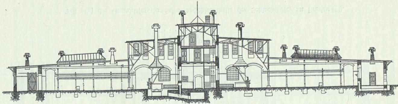
Querchnitt durch die Schlachthalle.
