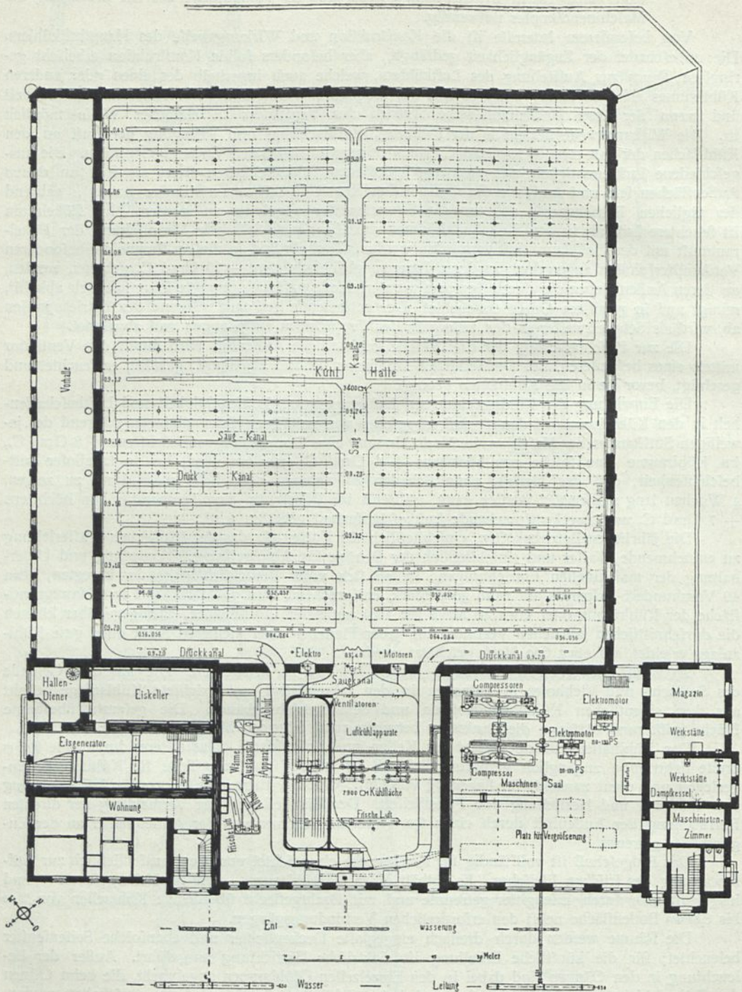
Grundriß des Kühlhauses im Schlachthof zu München 63) .
