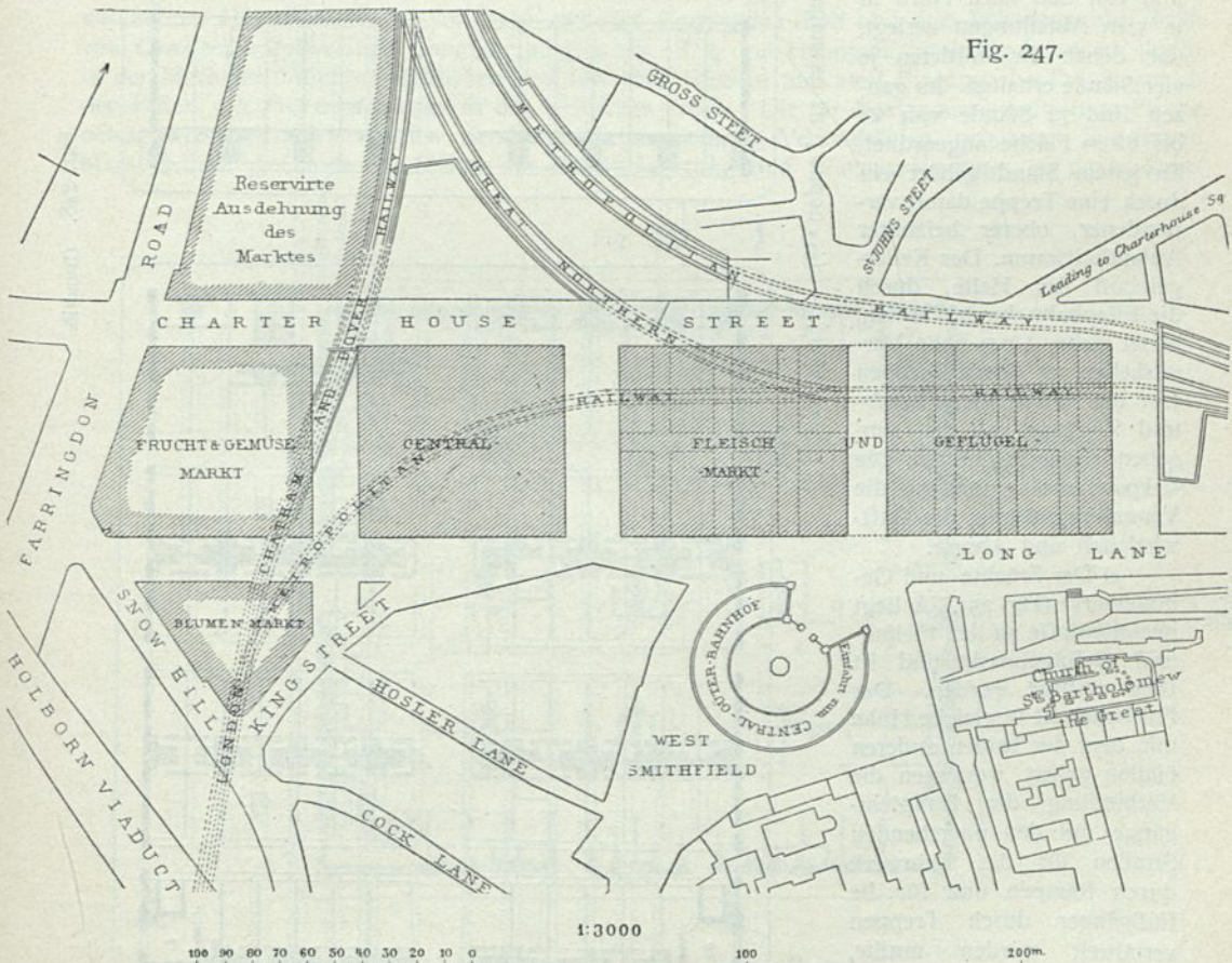
Lageplan der Smithfield-Märkte zu London 171) .
