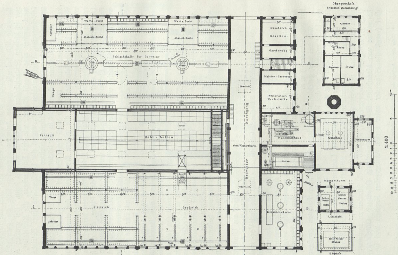
Grundriß des Hauptgebäudes im Schlachthof zu Guben.
