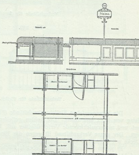
Stand für lebende Fische.
