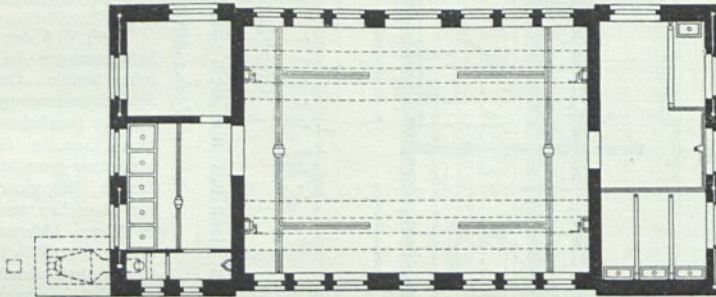
Grundriß.
