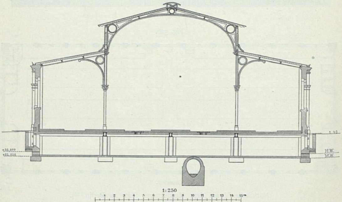
Querschnitt der Markthalle in Fig. 326.
