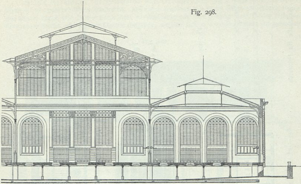
Zentralmarkthalle zu Florenz 204 ).
