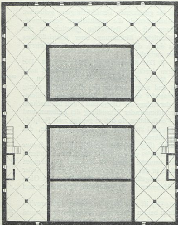
Fig. 270. Kellergeschoß.
