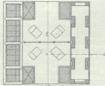
Verkaufsstand für Süßwasserfische
