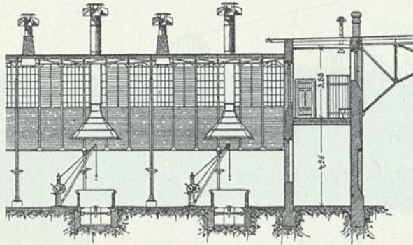
Teil des Längenschnittes durch den Brühräum.
