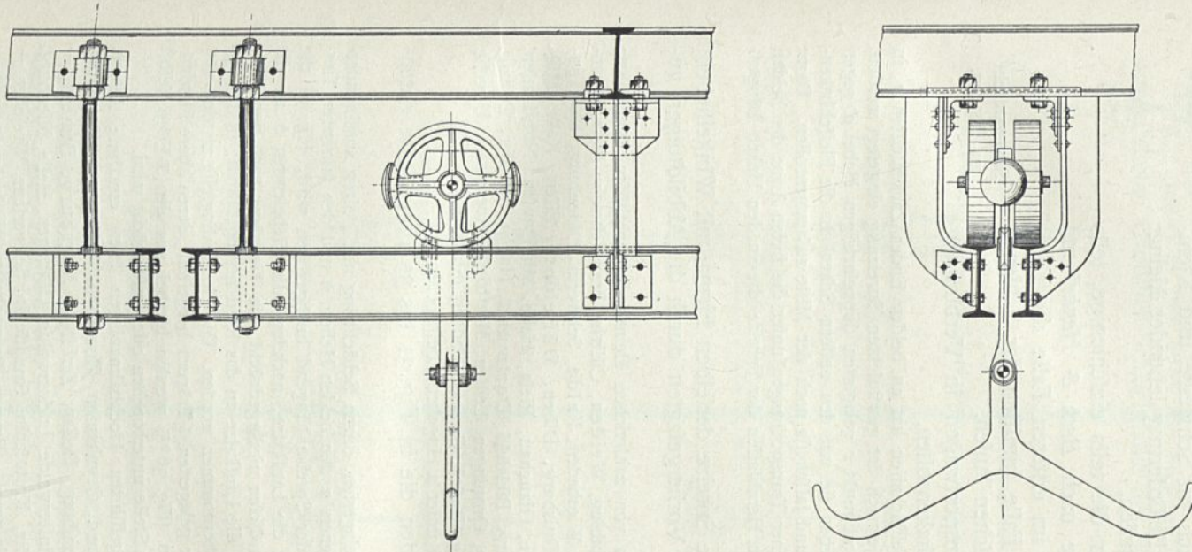
Transportwagen von Beck & Henkel [zu Kaffel.
