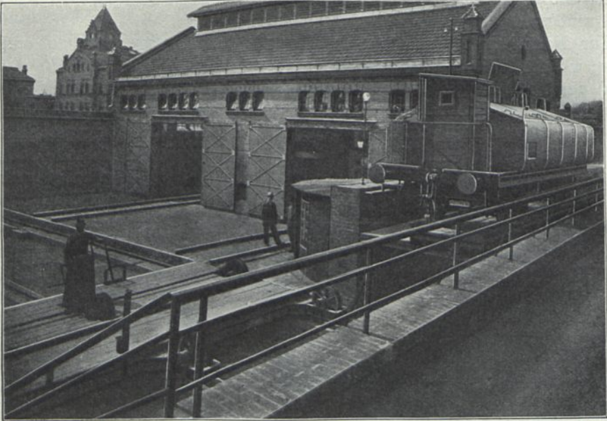
Hebevorrichtung der Eifenbahnwagen am Düngerhaus.
