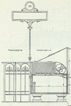
Standeinrichtung für Fische in der Großmarkthalle I zu Berlin 157) . 1/100 w. Gr.
