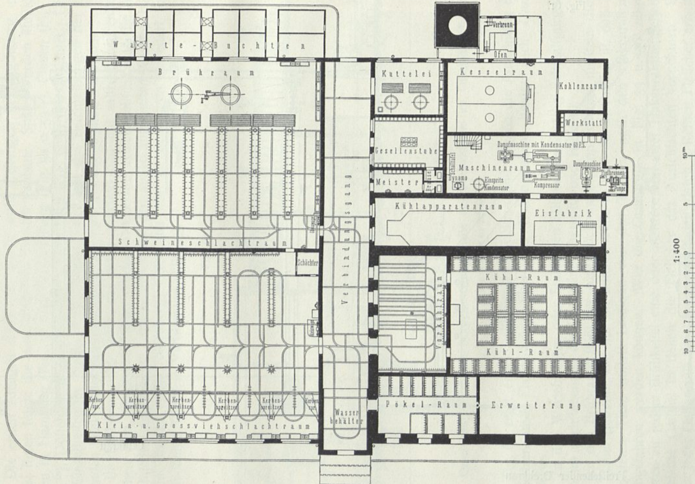
Grundriß des Hauptgebäudes auf dem Schlachthof zu Fulda 43) .
