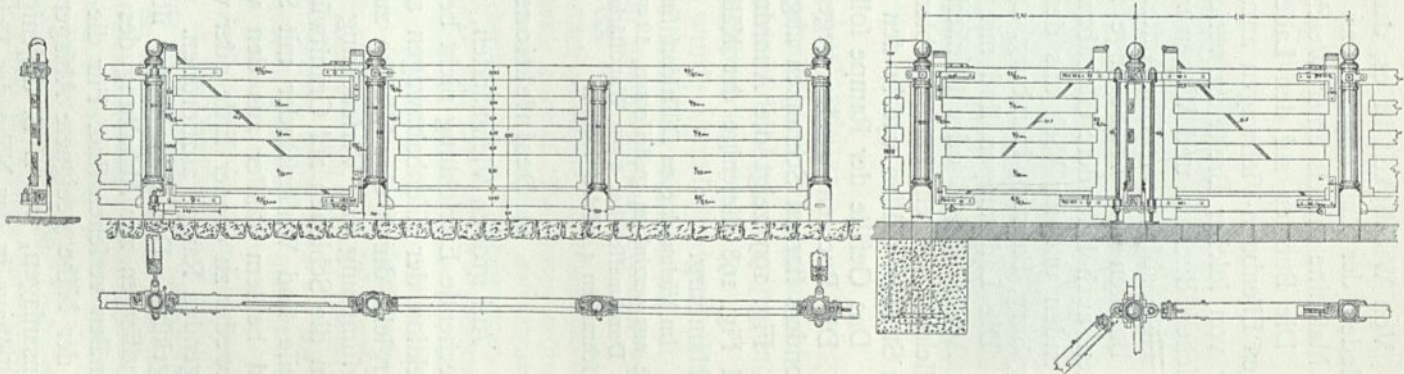
Schranken der Schweinebuchten in der Markthalle auf dem Viehhof Sternfchanze (Hamburg 87).
