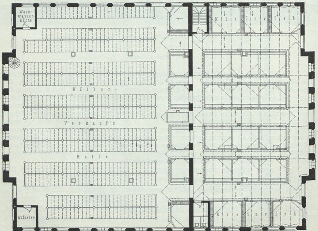
Kleinvieh-Markthalle auf dem Viehhof zu Düffeldorf 39) .
