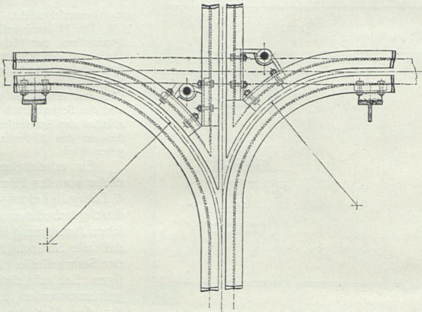
Doppelte Weiche der Transportgleise von Beck & Henkel zu Kassel.
