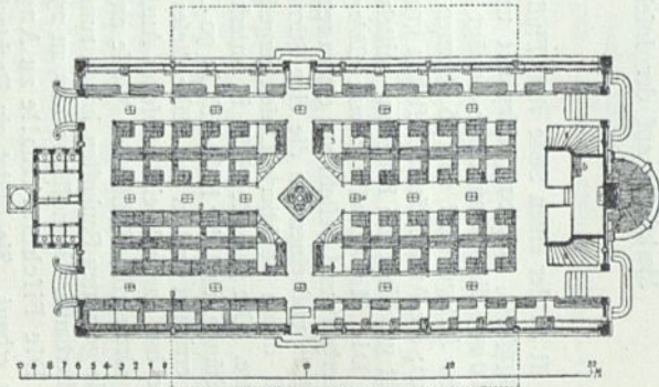
Markthalle Santa Chiara zu Grenoble 197).
