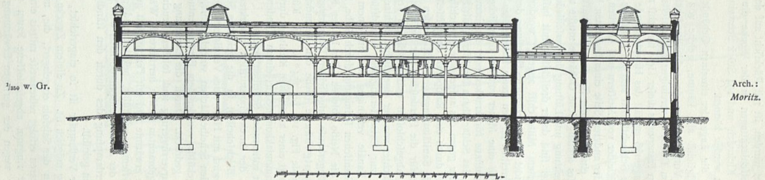
Längenschnitt durch die Großvieh- und Kleinvieh-Schlachthalle, sowie durch die Kuttelei.
