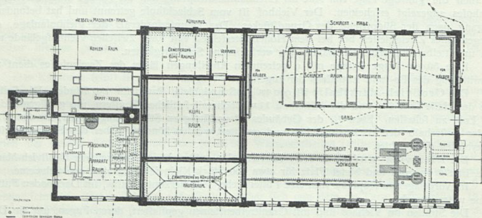
Hauptgebäude auf dem Schlachthof. - 1/500 w. Gr. Vom Schlacht- und Viehhof zu Landau 15).
