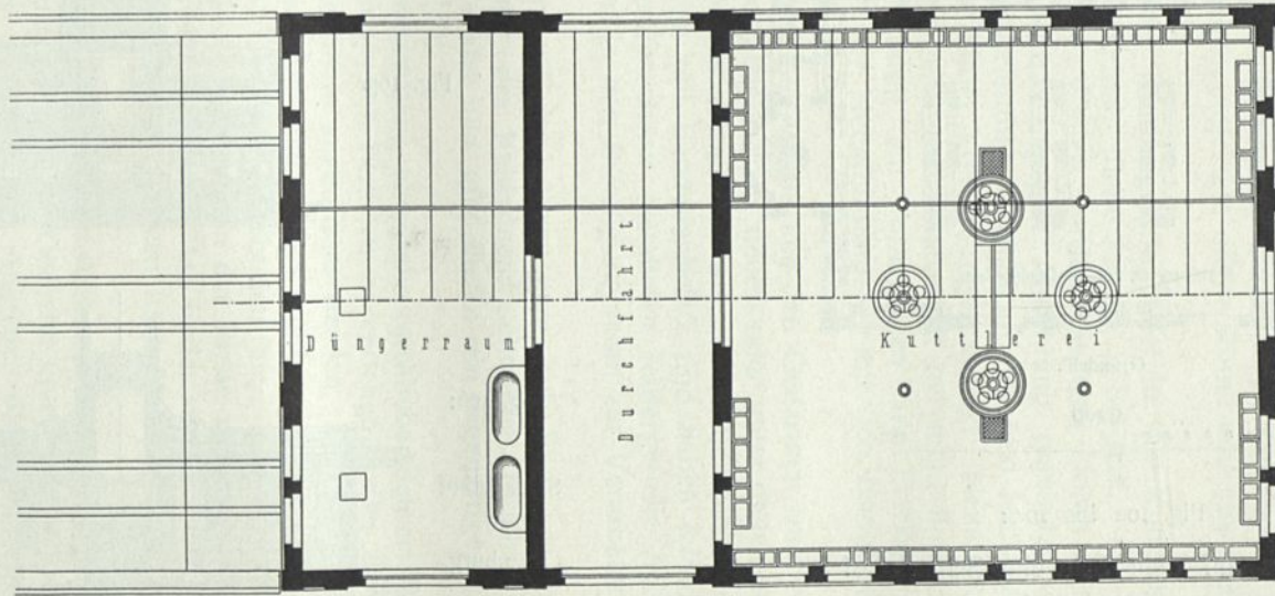
Kuttlei und Düngerhaus im Schlachthof zu Mannheim.
