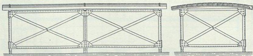
Schweine-Enthaarungstisch nach Moritz von Unruh & Liebig.
