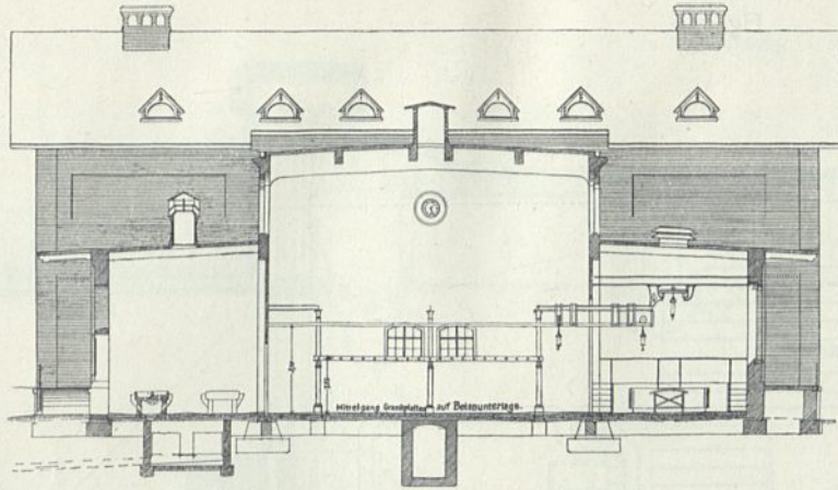
Querschnitt. — \frac{1}{300} w. Gr.
