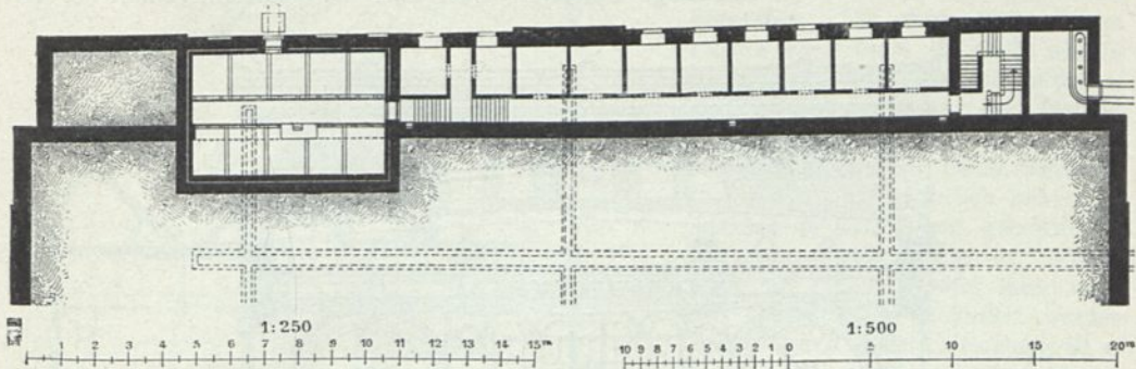
Fig. 317. Erdgeschoß.
