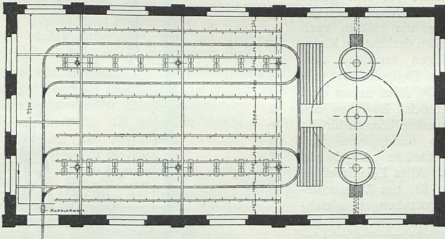
Grundriß.
