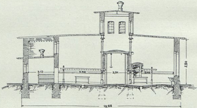
Querschnitt der Kleinvieh-Schlachthalle im Schlachthof zu Offenbach 36) .
