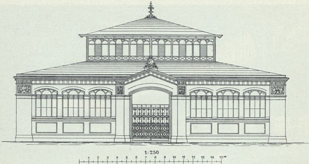
Seitenansicht der Markthalle in Fig. 326.
