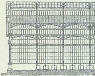
Fig. 276. Längenfchnitt 194) .
