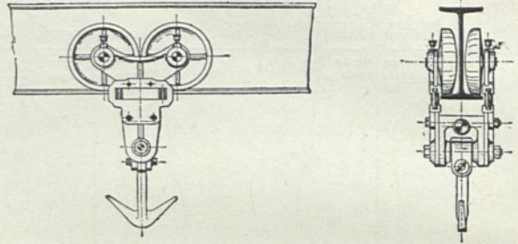
Transportwagen.
