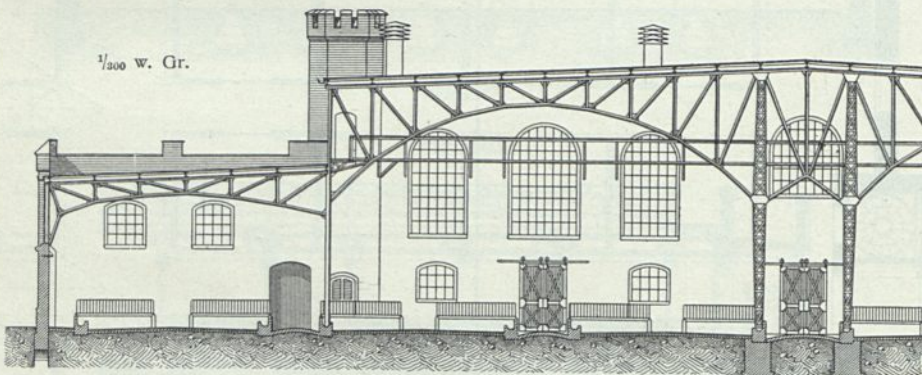
Querschnitt.
