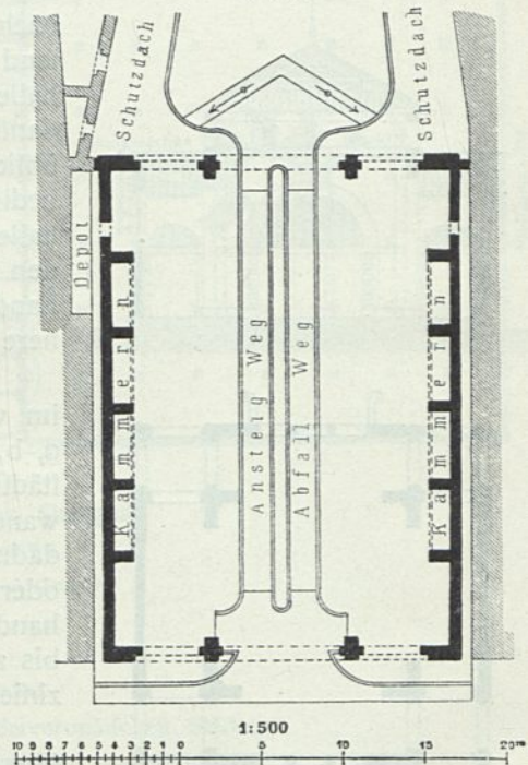
Getreidehalle zu Courtenay 256) .
