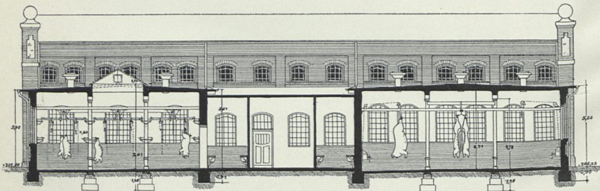
• SCHNITT E-F •
