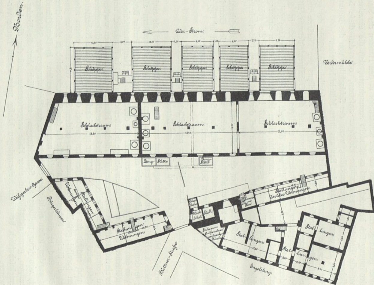
Lageplan des alten Schlachthofes zu Breslau 1) .
