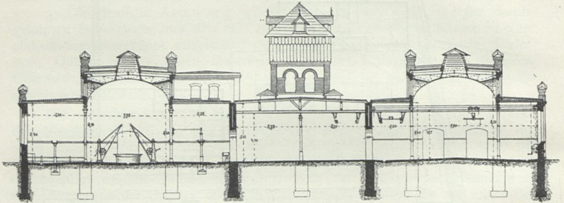
Querfchnitt durch das Hauptgebäude des Schlachthofes zu Guben 14) .
