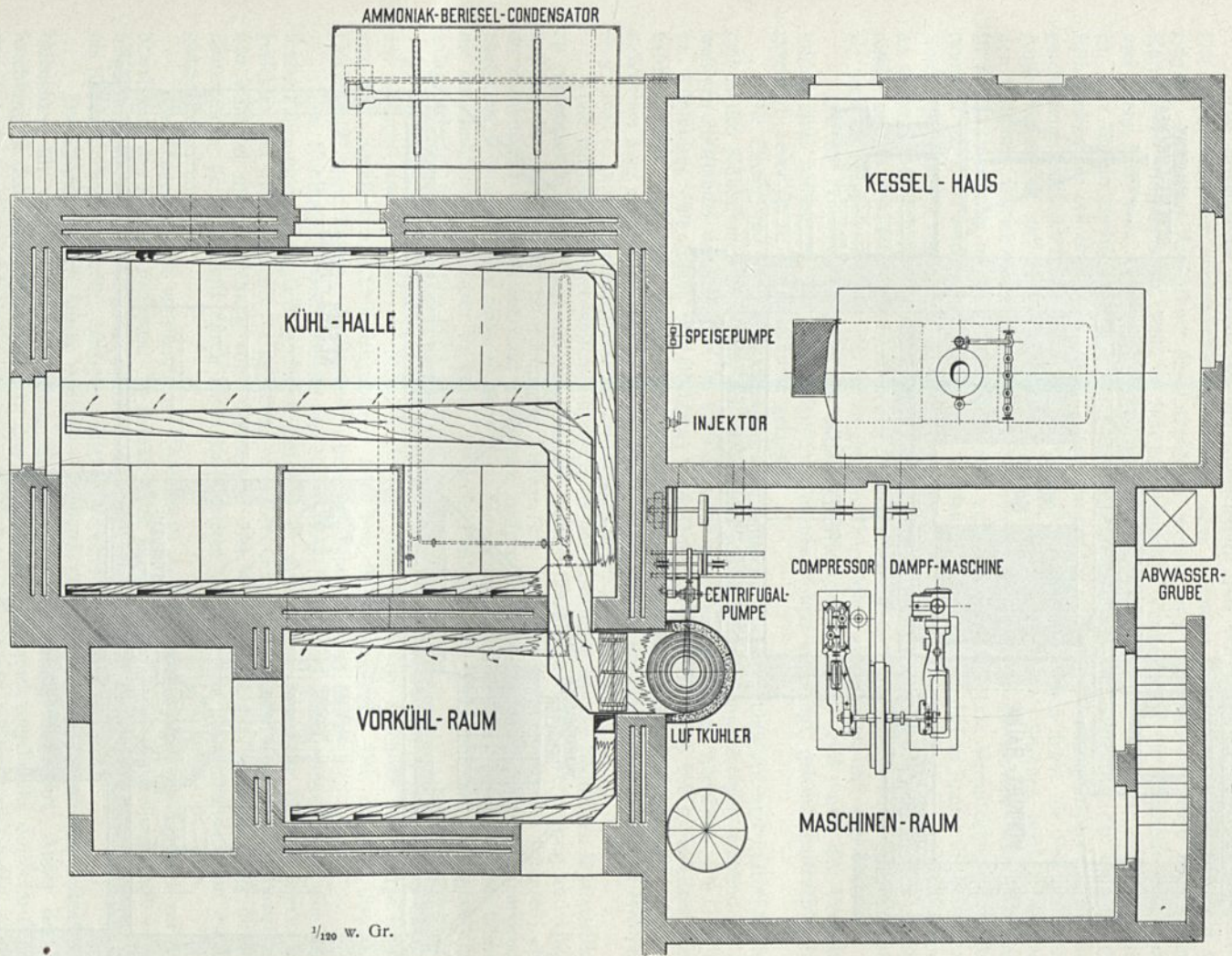
Grundriß.
