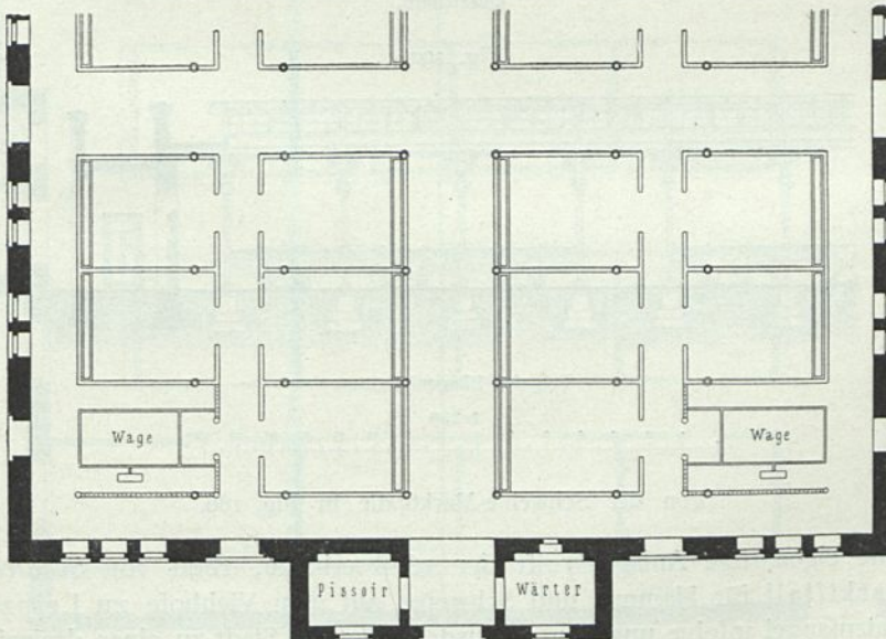
Teil des Grundriffes. - \frac{1}{200} w. Gr.
