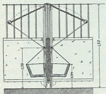
Querschnitt.
