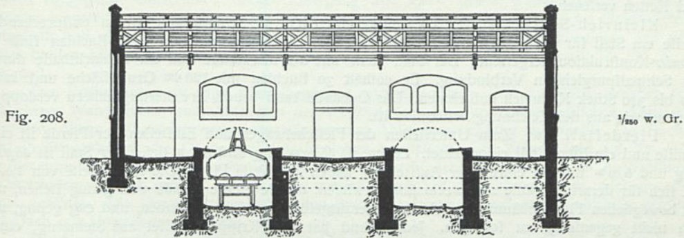
Längenschnitt durch das Düngerhaus des Schlachthofes zu Barmen 112) .
