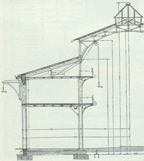
Querschnitt zu Fig. 355 242) .
