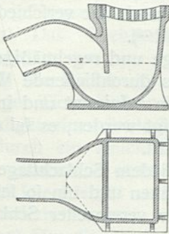
Einlauf in den Hallen und Ställen.
