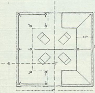
Verkaufsstand für Seefische in den Zentralhallen zu Paris 158) .
