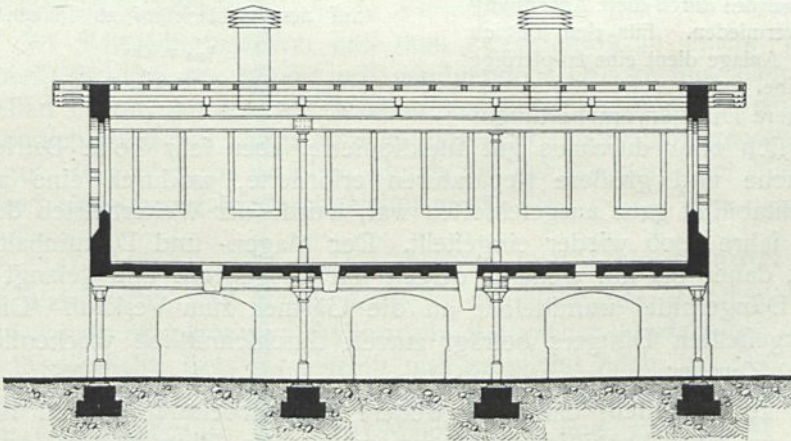
Längenschnitt.
