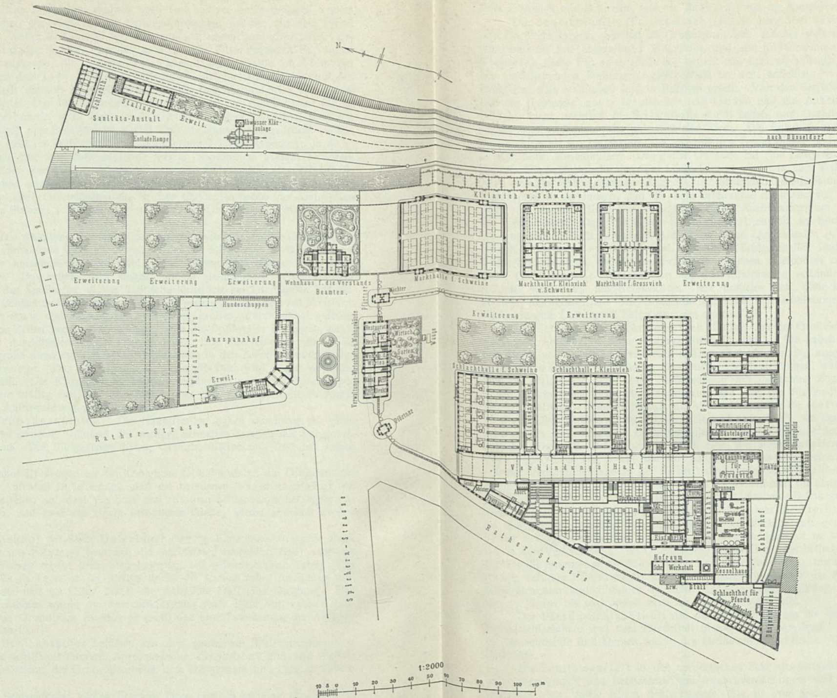
Schlachthof und Viehmarkt zu Düsseldorf.
