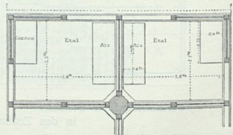
Stand für Kleinverkauf in den Zentralhallen zu Paris 160) .
