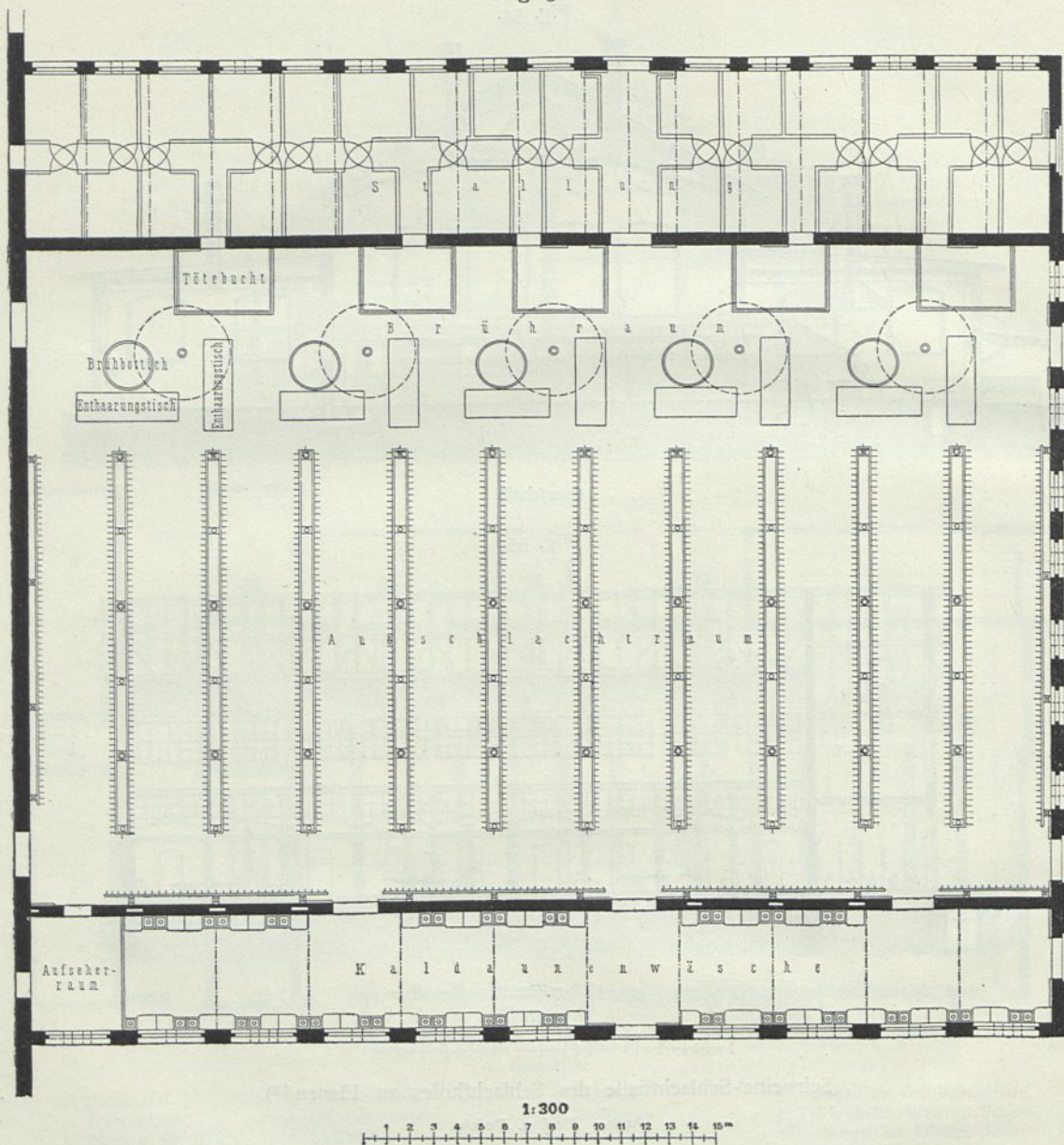
Schweine-Schlachthalle des Schlachthofes zu Düffeldorf 39) .
