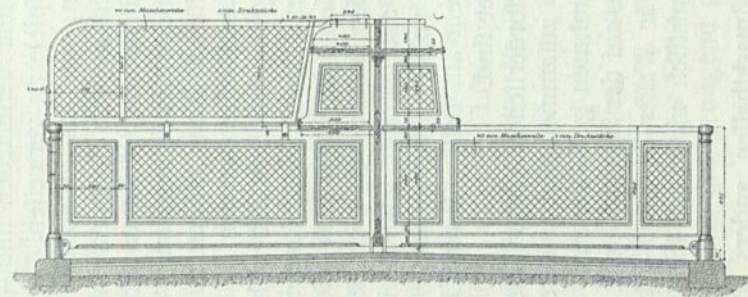
Standeinrichtung für Fleisch, Wild und Geflügel Gemüse, Obst, Mehl und Vorkoft in der Großmarkthalle I zu Berlin 156) .
