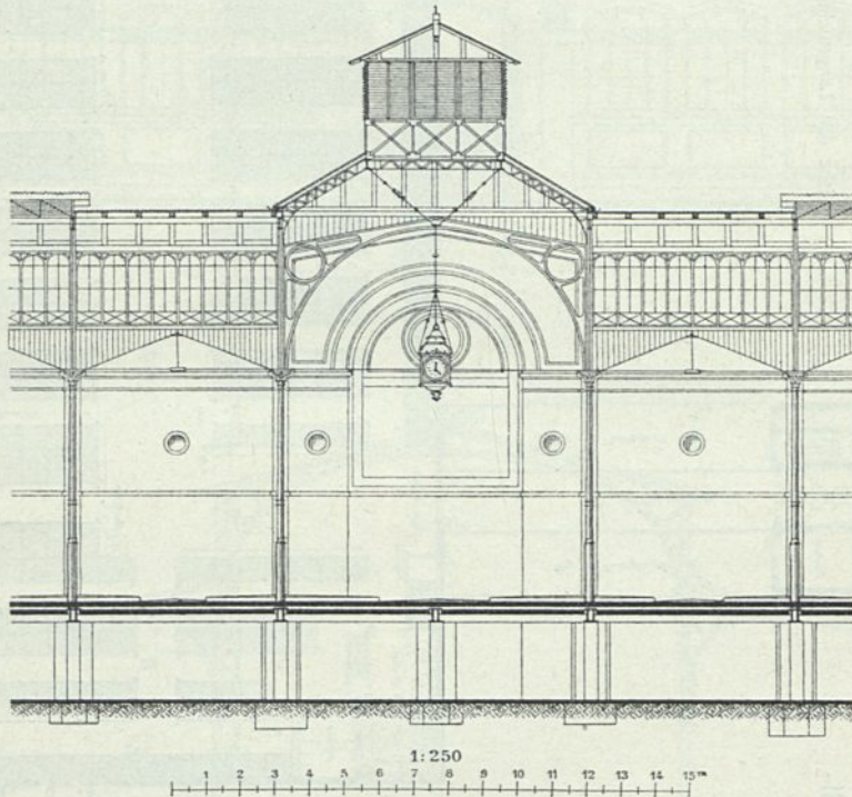
Langenschnitt zu Fig. 329 221 ).
