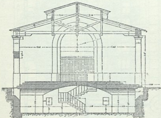
Querschnitt der Markthalle zu Nancy 196) .
