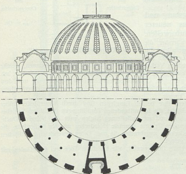
Halle aux blés zu Paris 257 .
