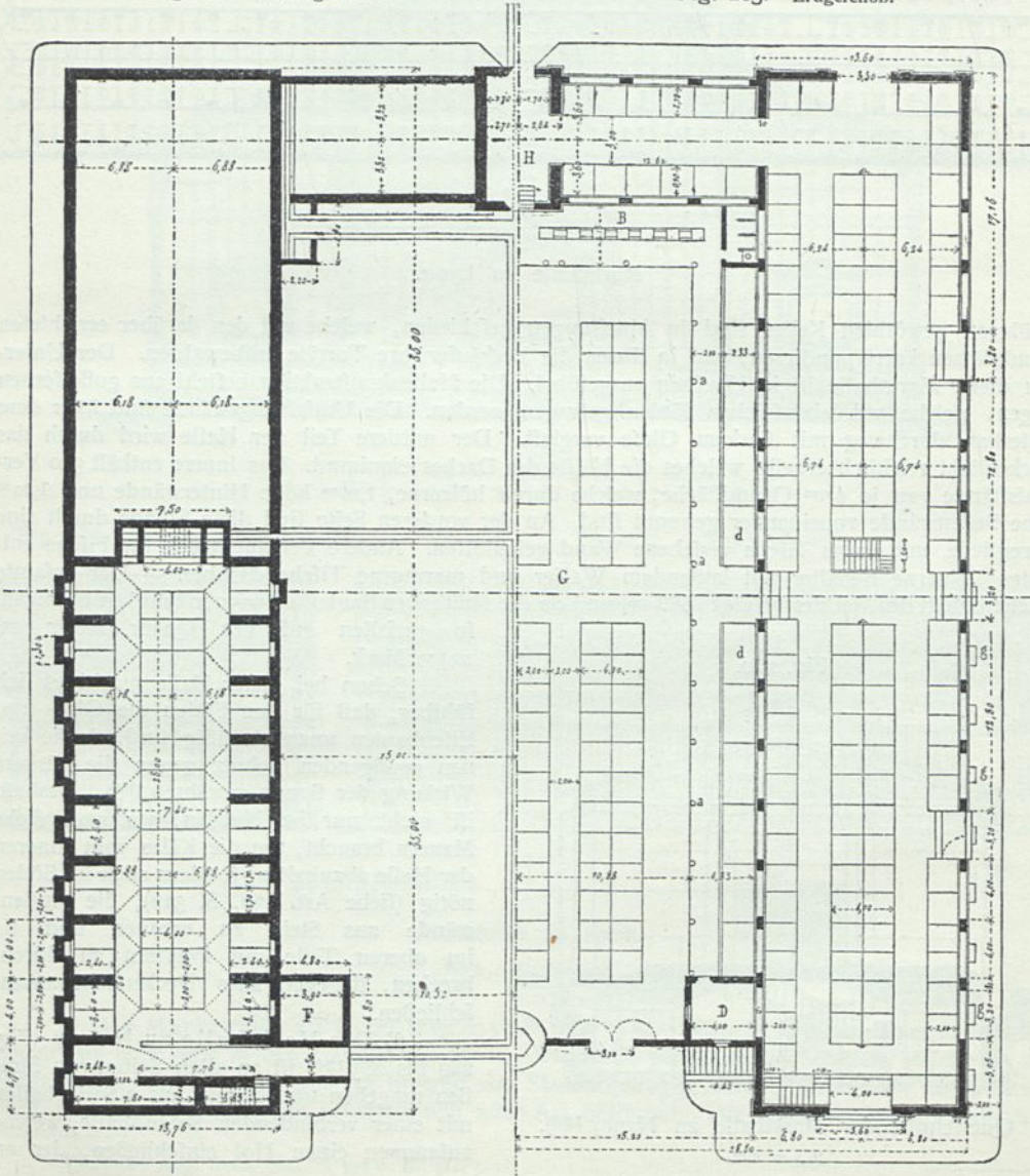
Markthalle zu Nancy 106 ). Arch.: Morey.
