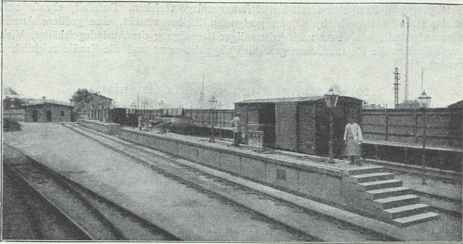
Desinfektionsanlage für Eisenbahnwagen auf dem Viehhof zu Leipzig 32) .
