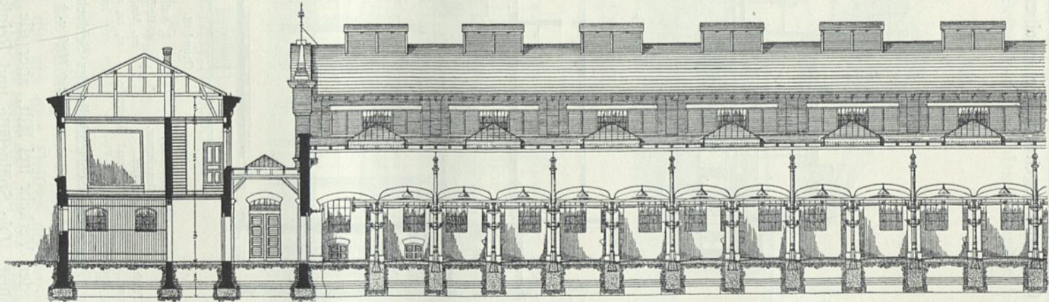
Längenschnitt.
