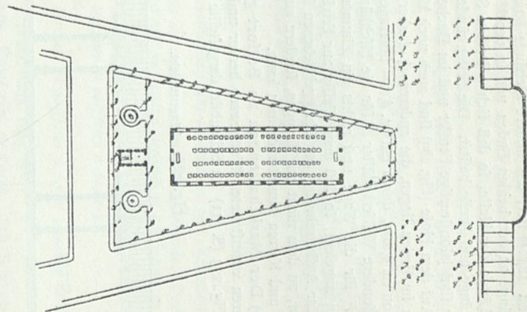
Fischmarkthalle zu Angers 197).
