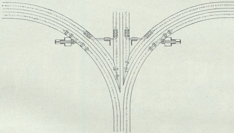
Doppelte Weiche für Hochbahngleise nach Kaiser & Co. zu Kassel.
