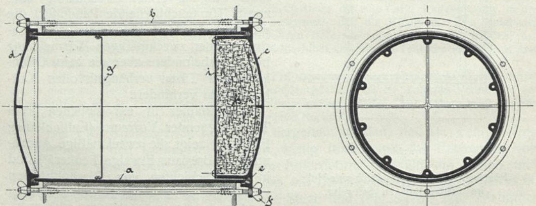
Lüftungsrohr für Kühlhäuser nach Schwarz.
