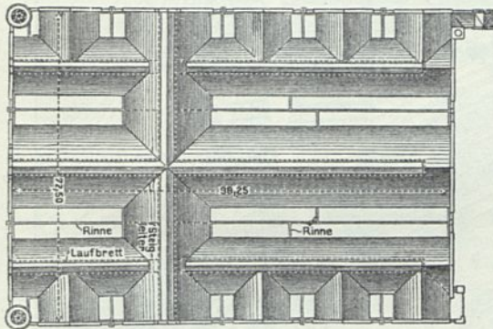
Hauptmarkthalle zu Cöln. Dachanordnung 233 ).
