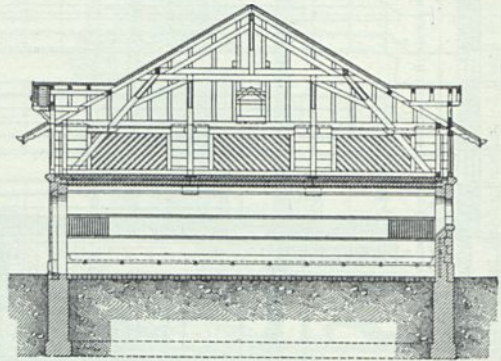
Querschnitt.
