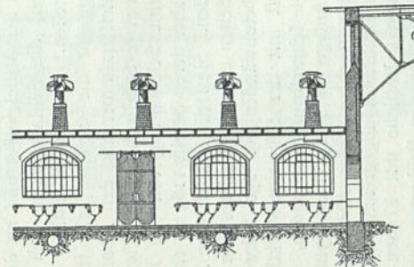
Teil des Längenschnittes durch die Kuttelei.
