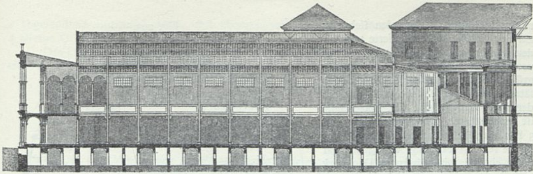
Fig. 291. Längenschnitt 199).
