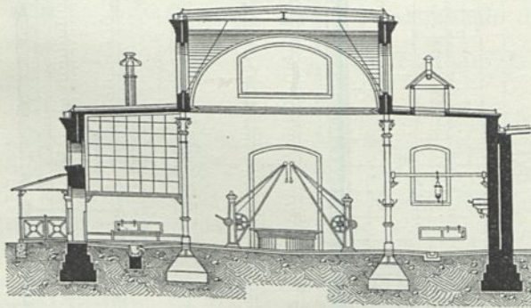
Querchnitt durch die Schweine-Schlachthalle des Schlachthofes zu Posen.
