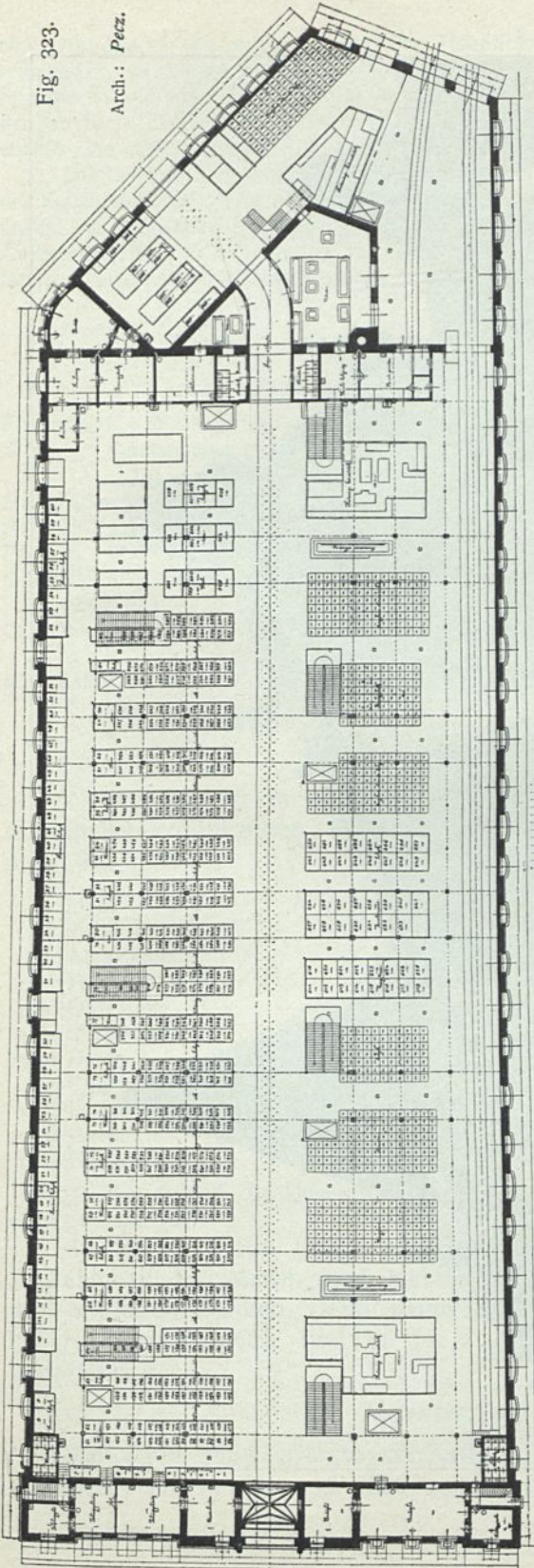
Grundriß der Zentralmarkthalle zu Budapest 217) .
