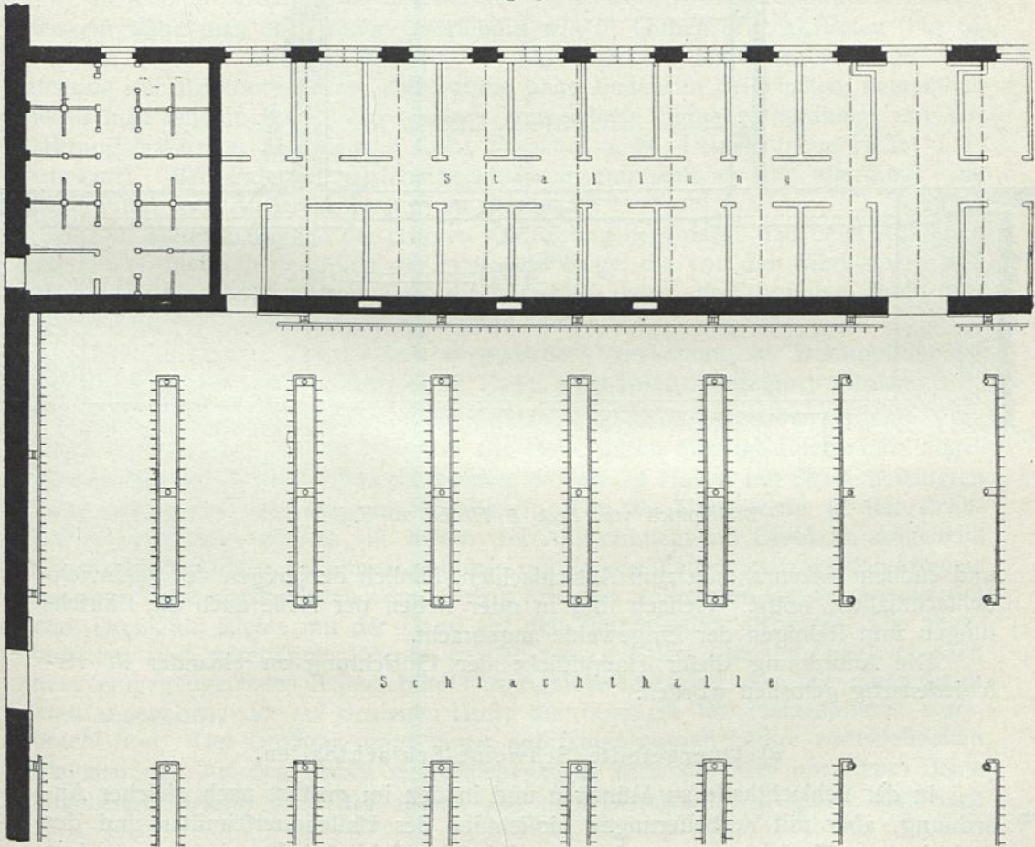
Grundriß.
