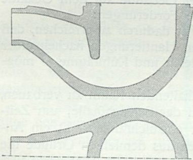
Straßeneinlauf.
