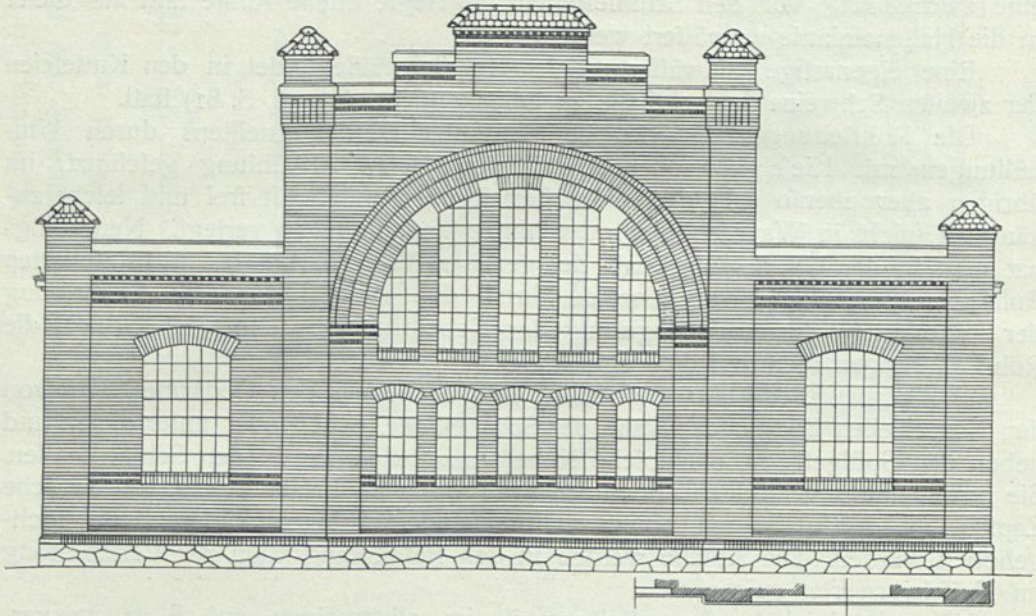
Giebelansicht. — \frac{1}{150} w. Gr.
