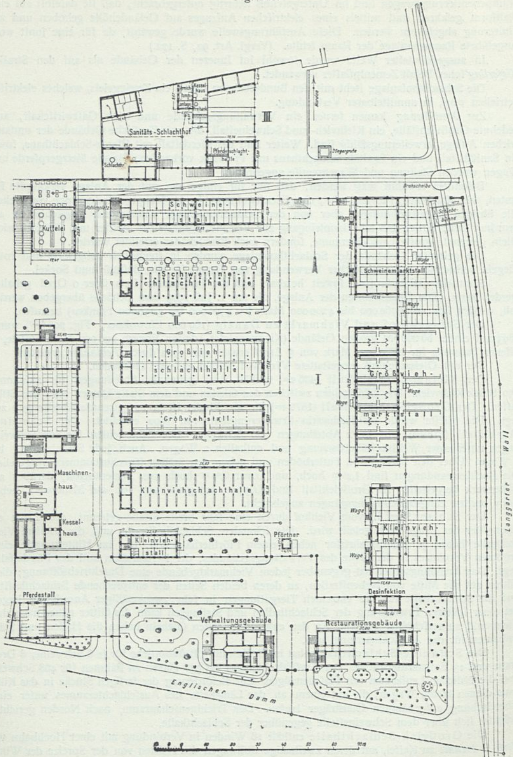
Schlachthof und Viehmarkt zu Danzig 110) .
