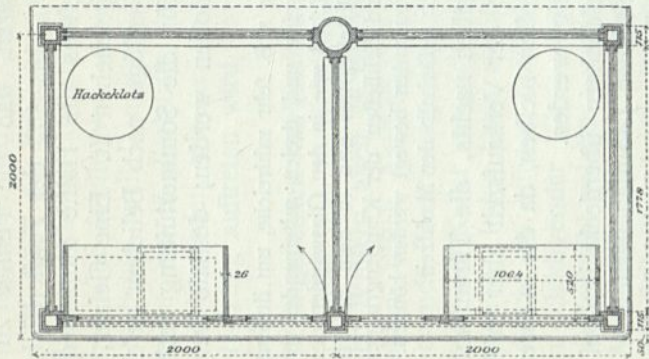
Standeinrichtung für Fleisch, Wild und Geflügel Gemüse, Obst, Mehl und Vorkoft in der Großmarkthalle I zu Berlin 156) .
