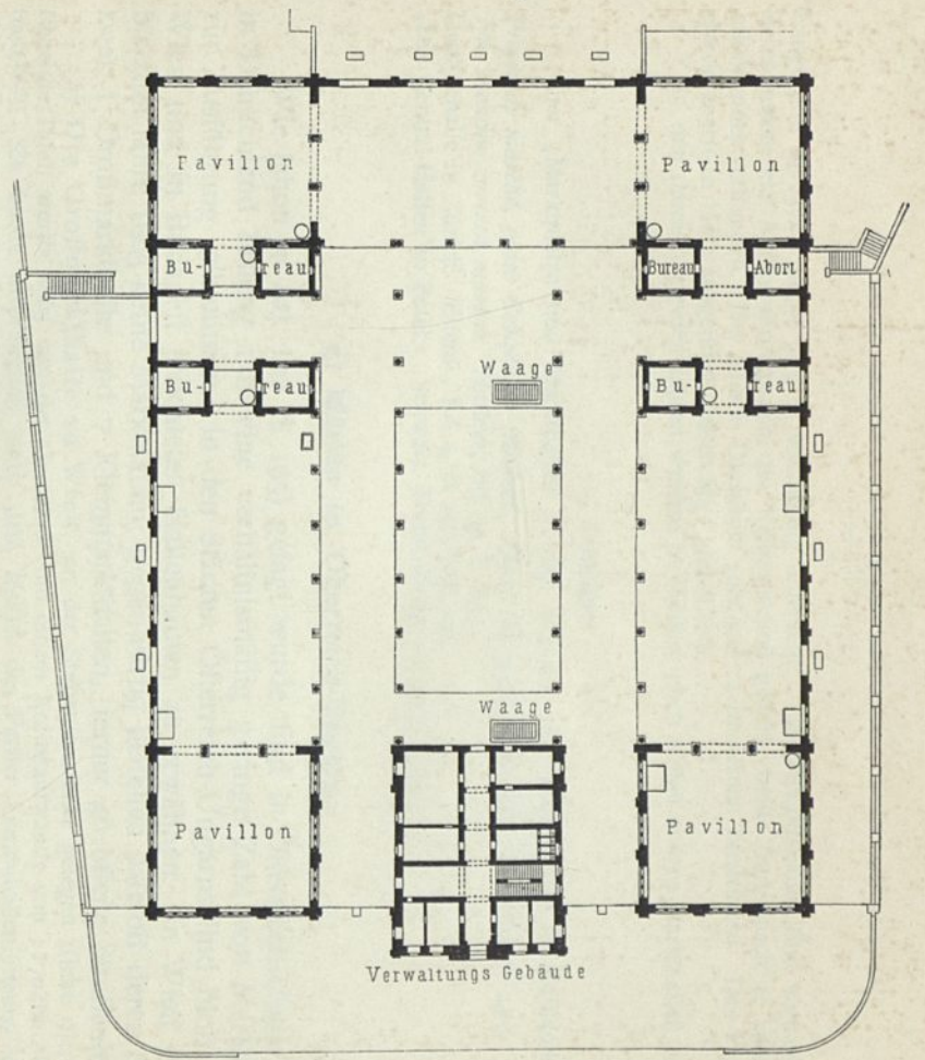
Grundriß des Erdgeschosses.
