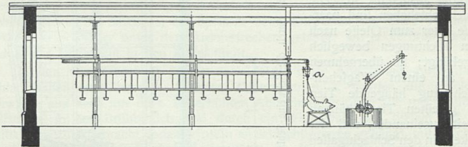
Längenschnitt.
