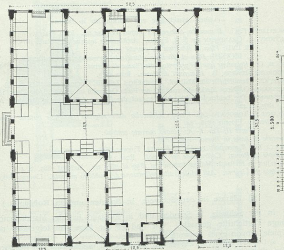
Grundriß.
