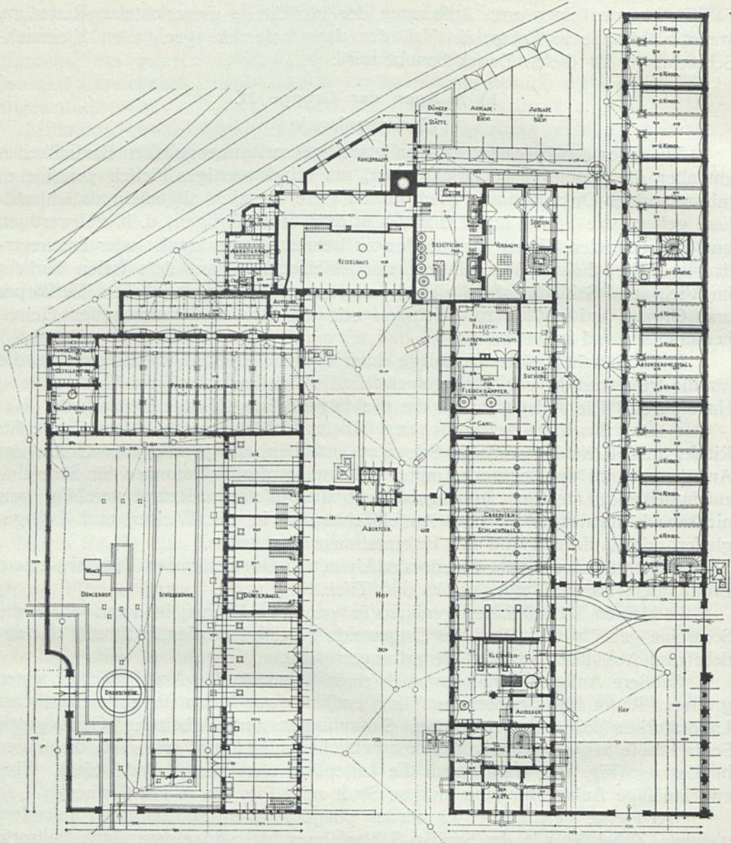
Sanitätsanlage auf dem Schlacht- und Viehhof zu Leipzig 64).
