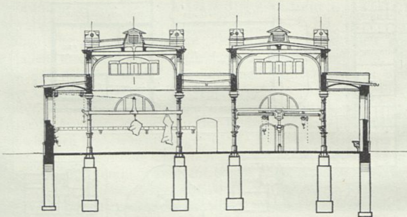
Querfchnitt durch den Schlachthallenbau zu Landau 15) .
