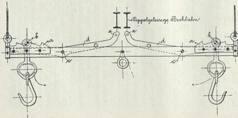
Kerbenfpreise mit Fleischhakenrollen
