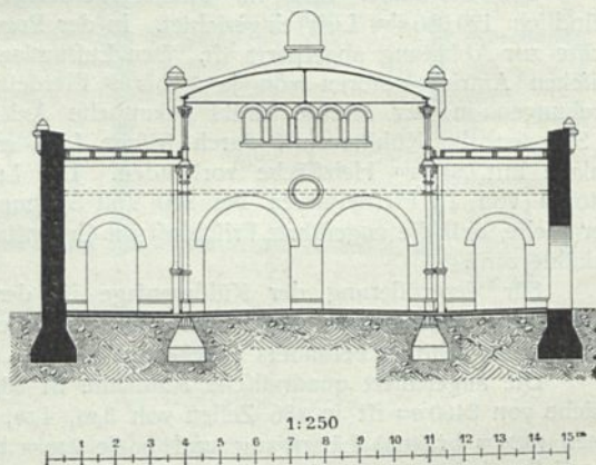
Querschnitt der Verbindungshalle im Schlachthof zu Pofen.
