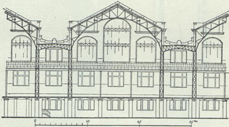
Querschnitt zu Fig. 332 u. 333 223) .
