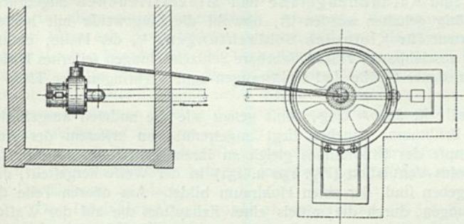
Grundriß.
