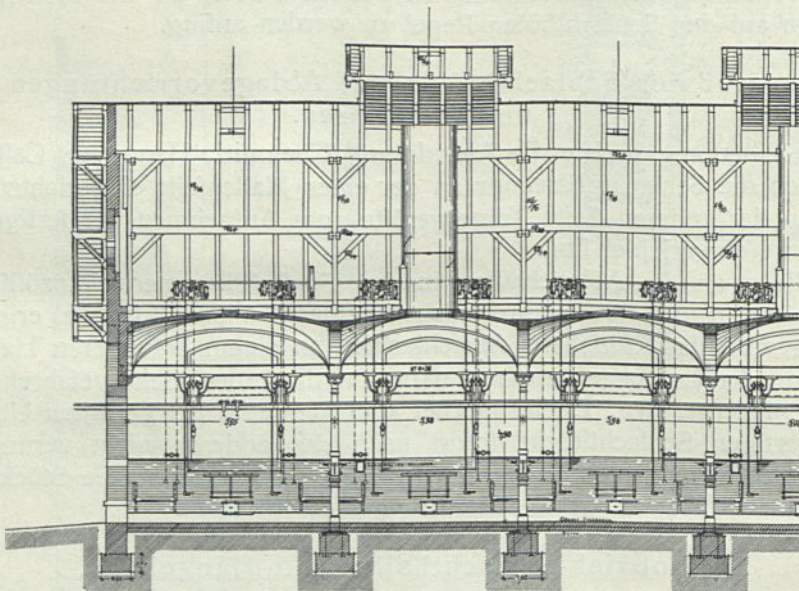
Längenschnitt.
