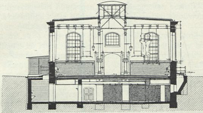
Querschnitt.
