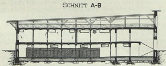
SCHNITT A-B
