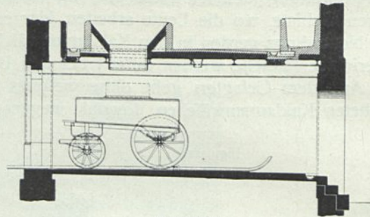
Querschnitt.
