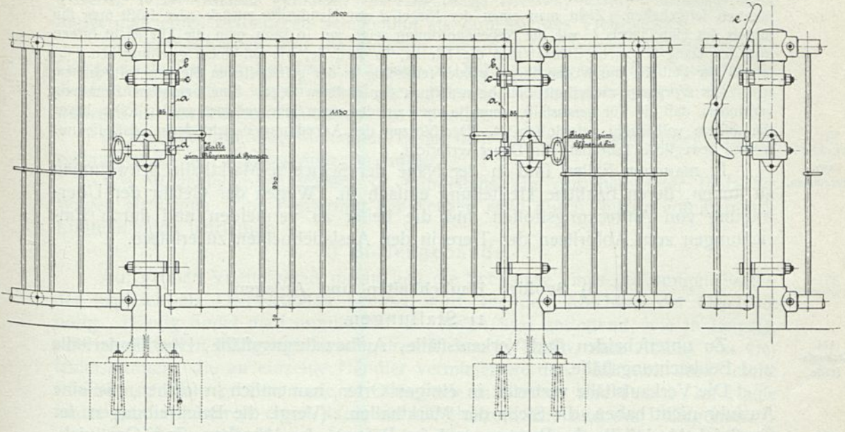
Anficht.
