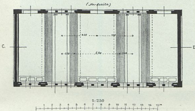
Grundriß des Düngerhauses im Schlachthof zu Barmen.
