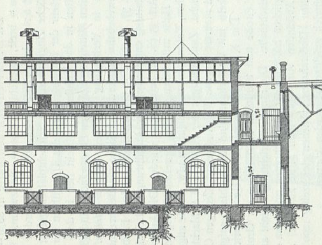
Teil des Längenschnittes durch den Mittelbau.
