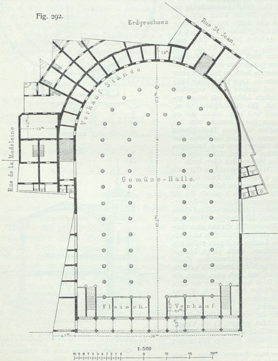
Markthalle Ste.-Madeleine zu Brüssel 200).
