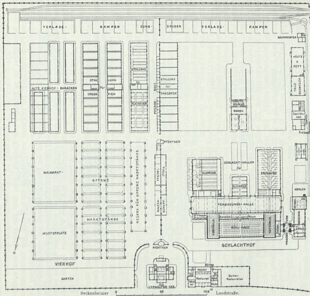
Schlachthof und Viehmarkt zu Mannheim 111) .
