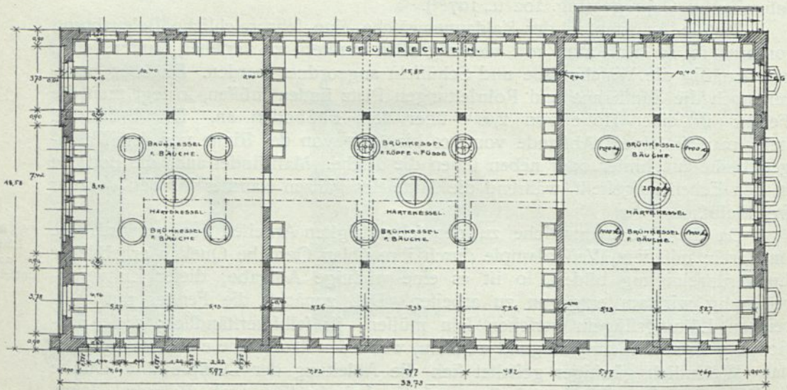
Grundriß. — \frac{1}{300} w. Gr.
