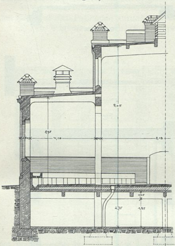
Querschnitt zu Fig. 107 u. 108 64 ).
