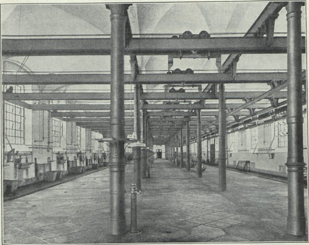
Innenansicht zu Fig. 16 u. 17 32) .
