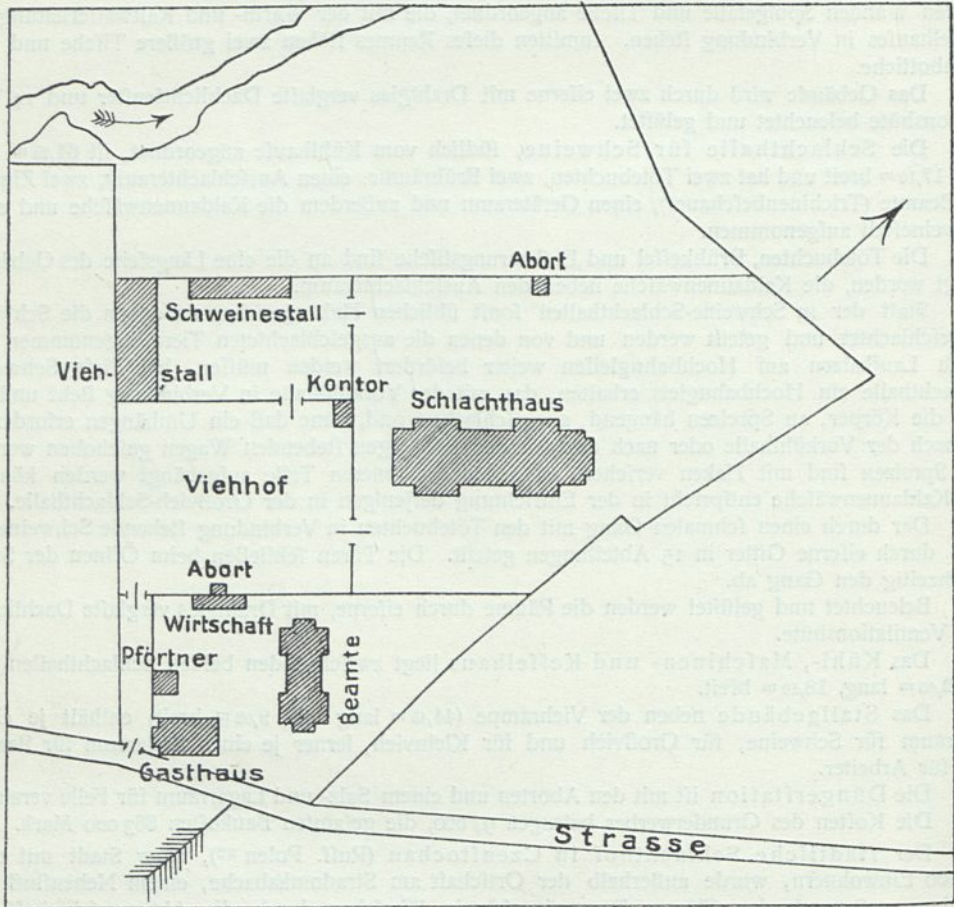
Schlachthof zu Czenftochau 92) .
