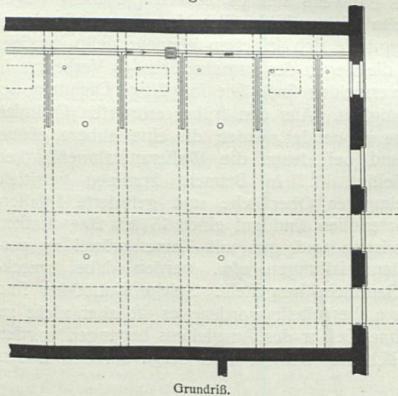
Großvieh-Schlachthalle auf dem Schlachthof zu Pofen. Arch.: Moritz.
