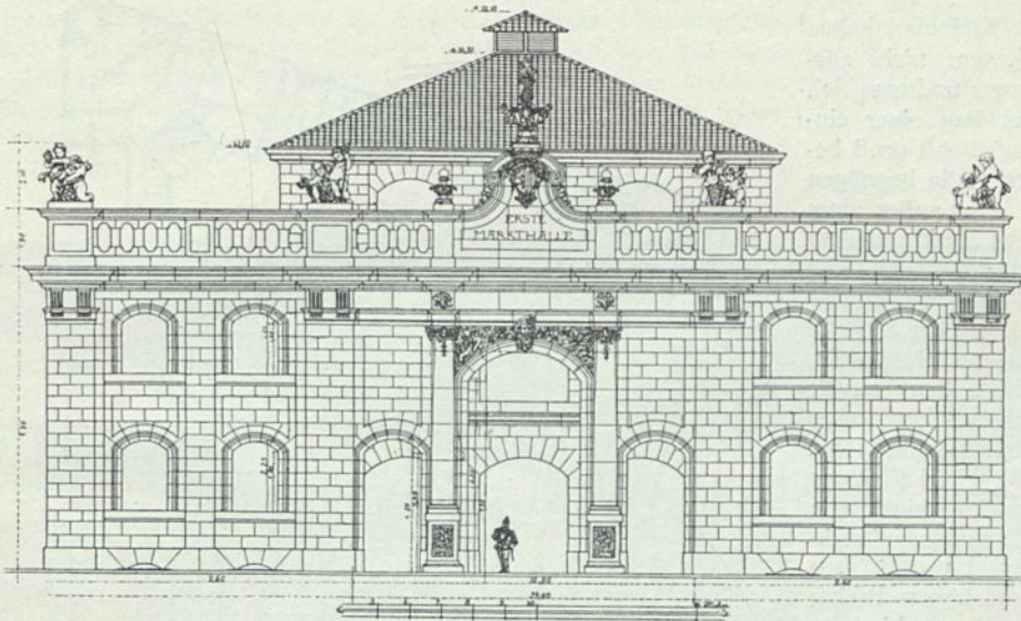
Anficht der Stirnseite.
