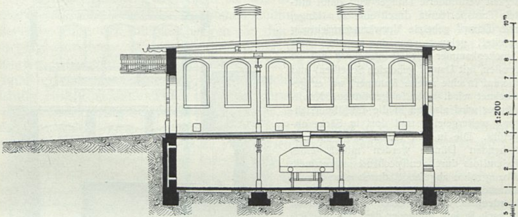
Querfchnitt.
