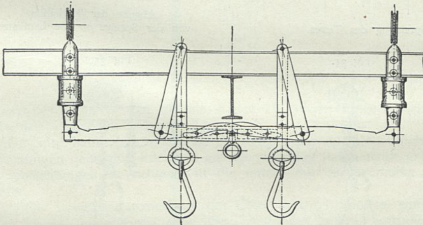
Fleischpreise mit Winkelhebeln von Beck & Henkel zu Kassel.
