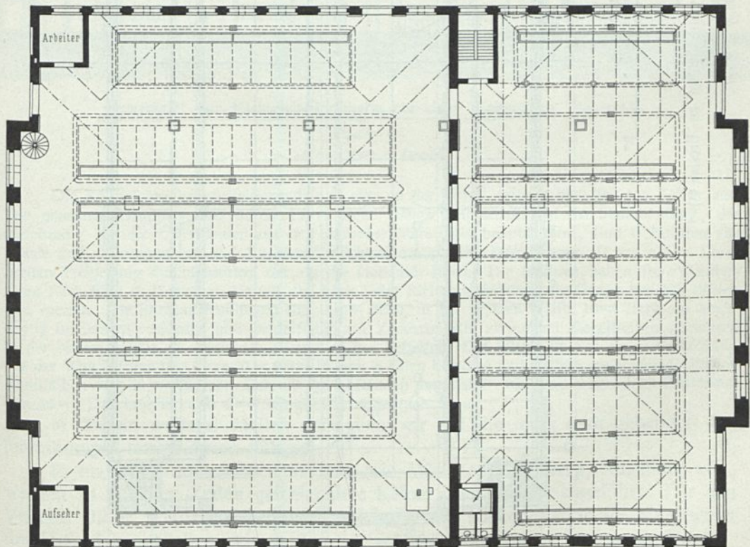
Großvieh-Markthalle auf dem Viehhof zu Düffeldorf 39) .
