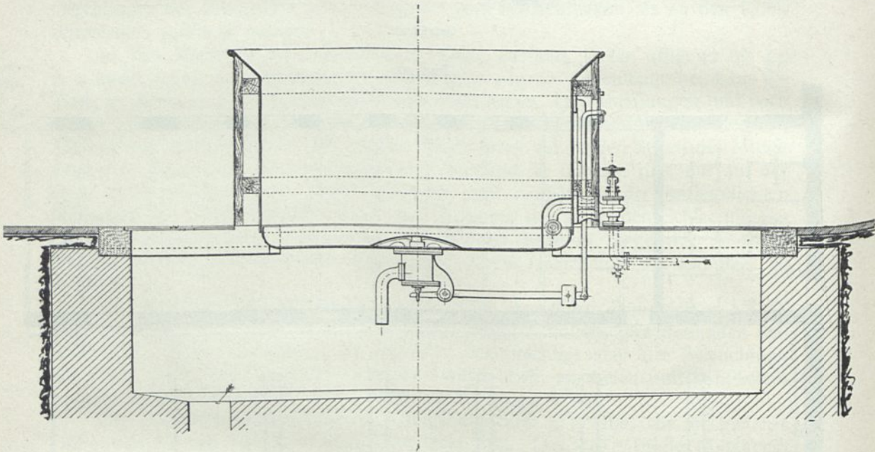
Brühbottich von Beck & Henkel zu Kassel 34) .
