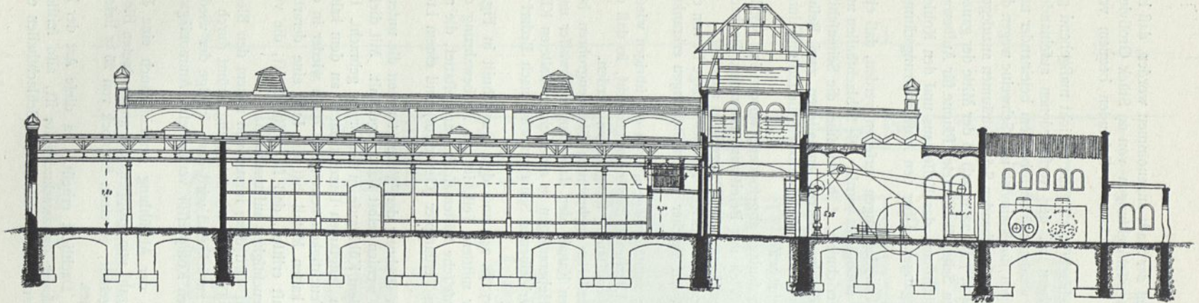
Längenschnitt durch die Kühlanlage.
