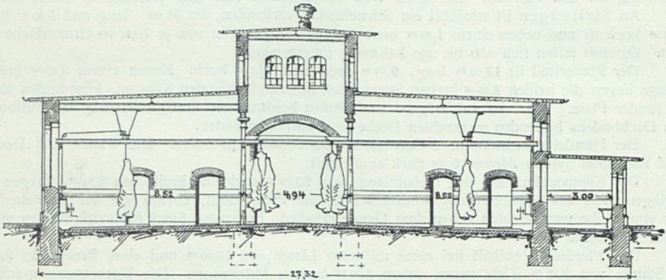
Querschnitt der Großvieh-Schlachthalle auf dem Schlachthof zu Offenbach a. M. 89).
