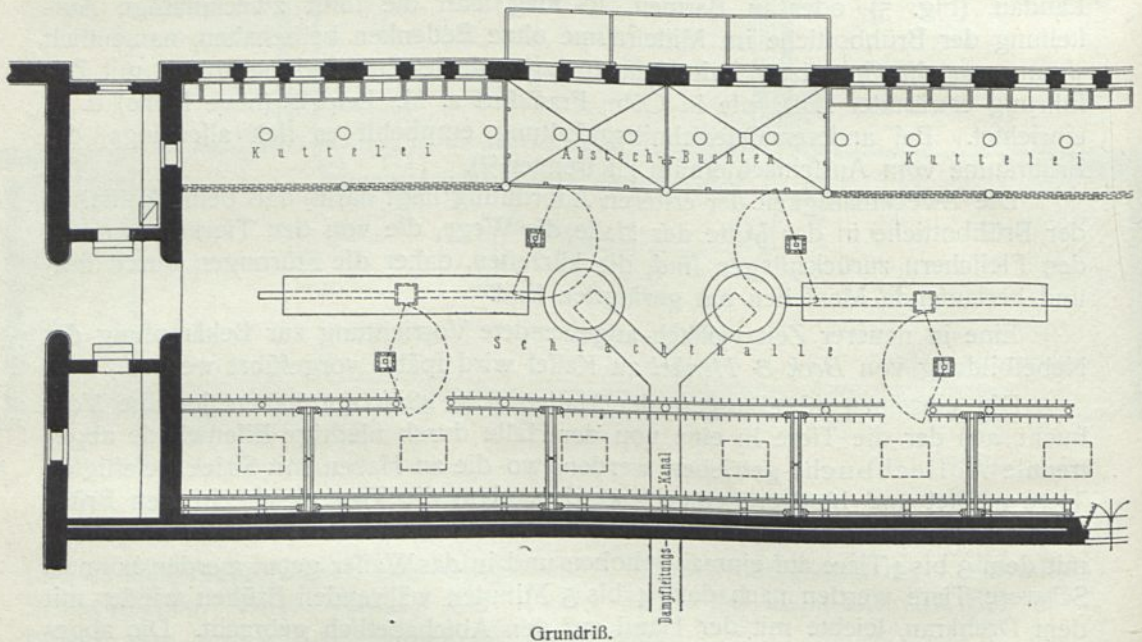
Grundriß.
