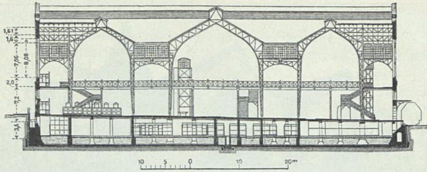
Querschnitt nach d d.
