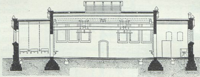
Längenschnitt.
