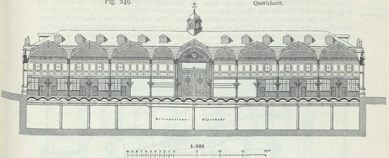
Fleischmarkt zu London 174).
