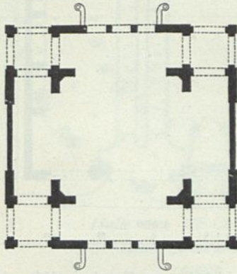
Getreidehalle zu Bréhal 255) .
