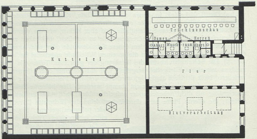
Grundriß.
