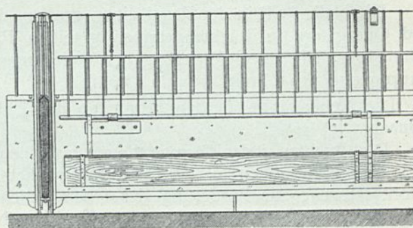
Längsschnitt.
