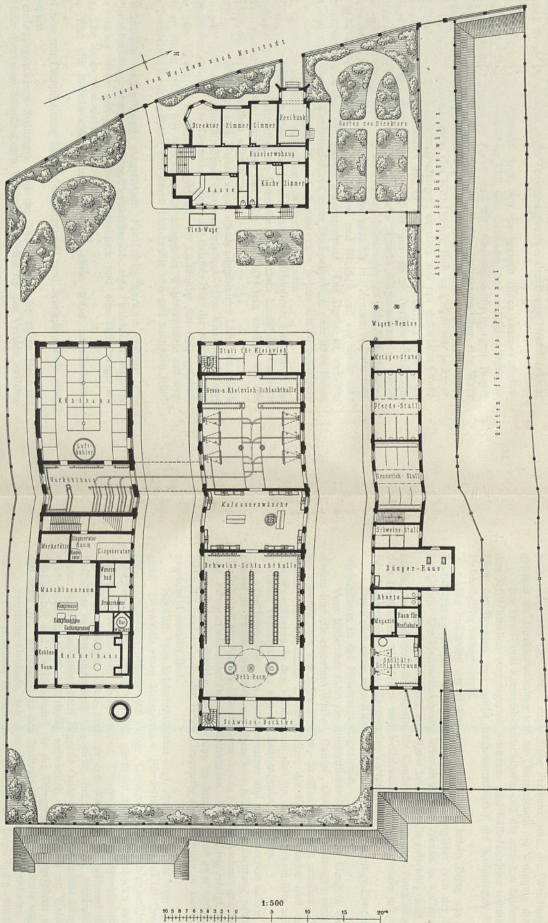
Schlachthof zu Weiden.
