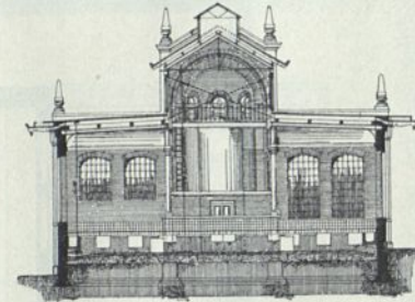
Längenschnitt.
