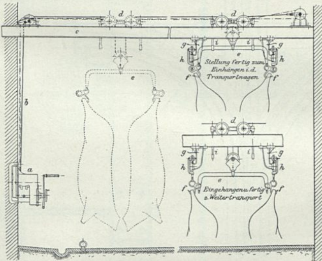
Einrichtungen der Hängebahn in Großvieh-Schlachthallen nach Moritz und Unruh & Liebig.
