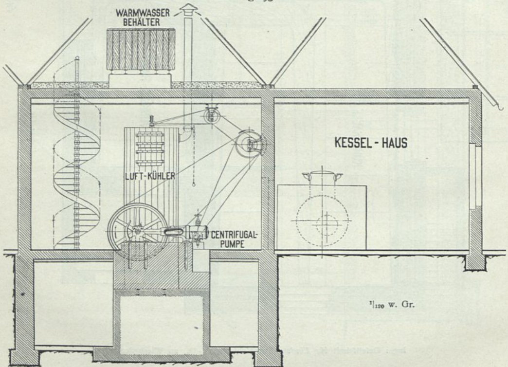
Querschnitt durch die Maschinenanlage Fig. 91 u. 92.
