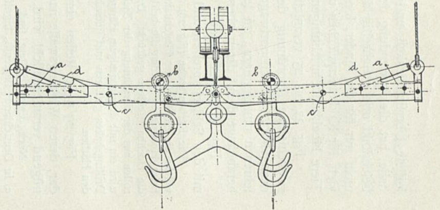
Kerbenfpreise mit Fleischhakenrollen
