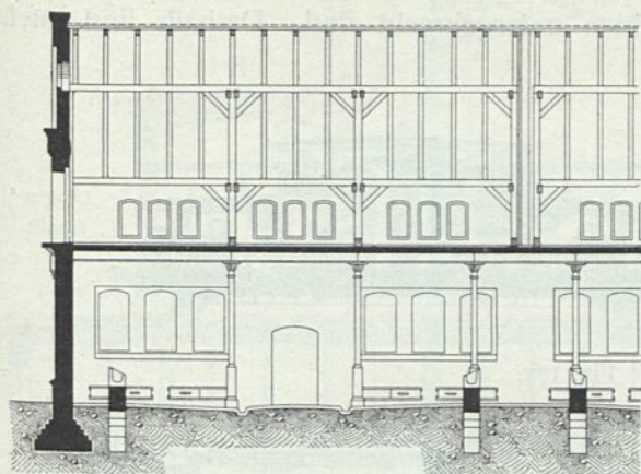
Teil des Längenschnittes.
