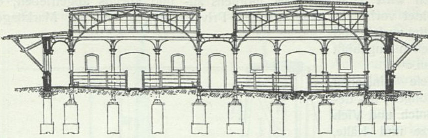
Querschnitt.
