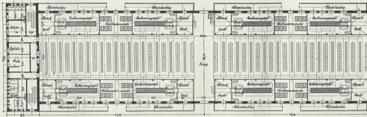
Grundriß. — \frac{1}{1000} w. Gr.
