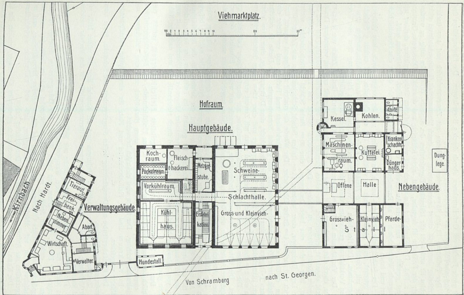
Schlachthof zu Schramberg 82 ).
