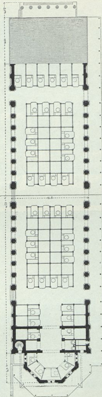
Fig. 309. Grundriß.
