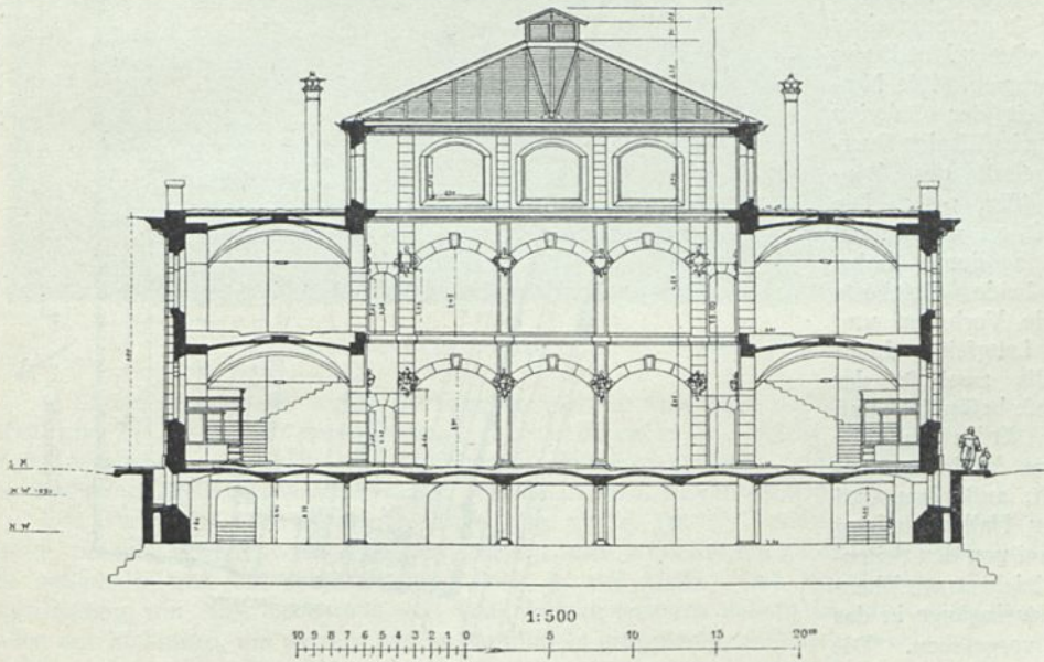
Querschnitt.
