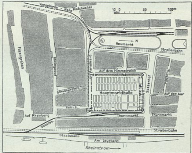
Neue Hauptmarkthalle zu Cöln. Lageplan 233) .
