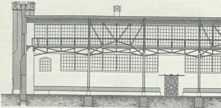
Längenschnitt.
