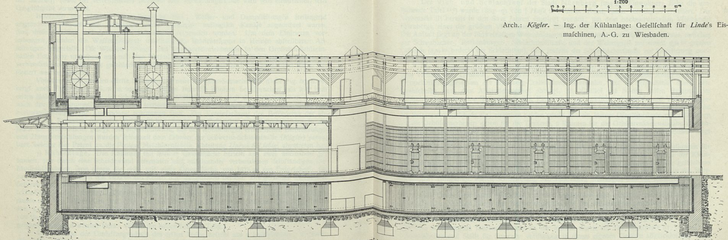
Längenschnitt.
