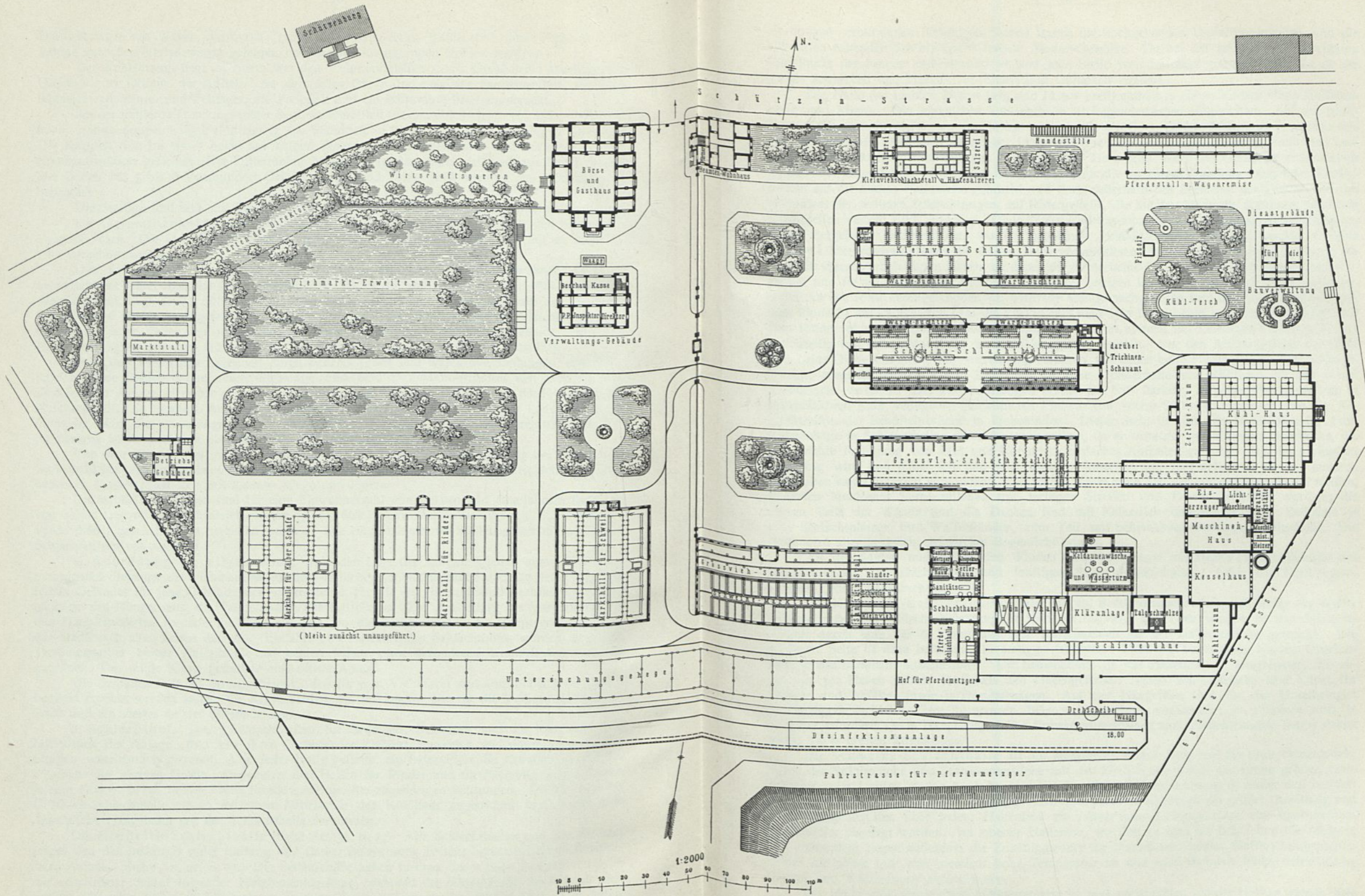
Schlachthof und Viehmarkt zu Barmen.
