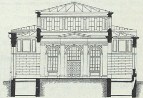
Fig. 319. Querschnitt durch die Halle.
