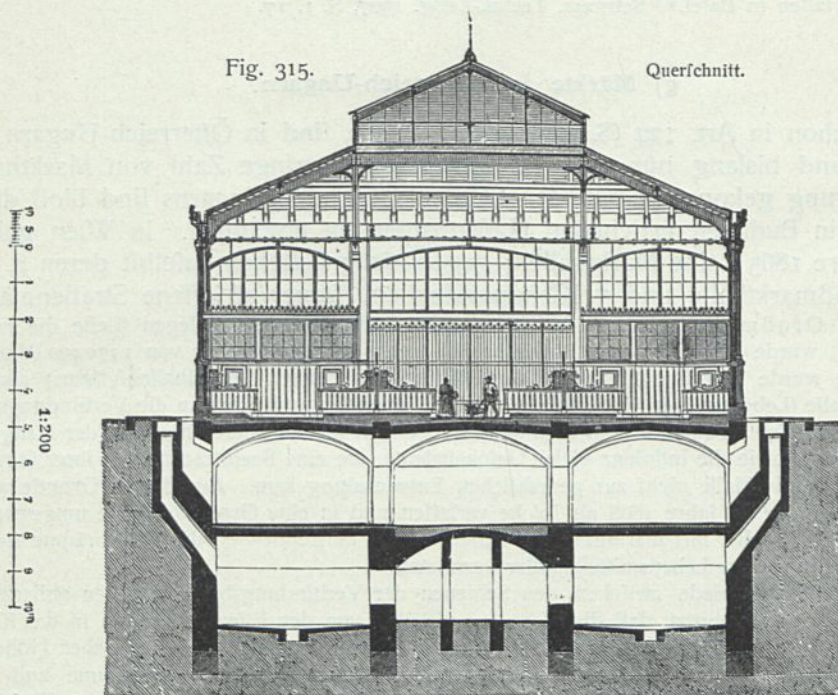
Kleinmarkthalle an der Stubenbastei zu Wien 215) .
