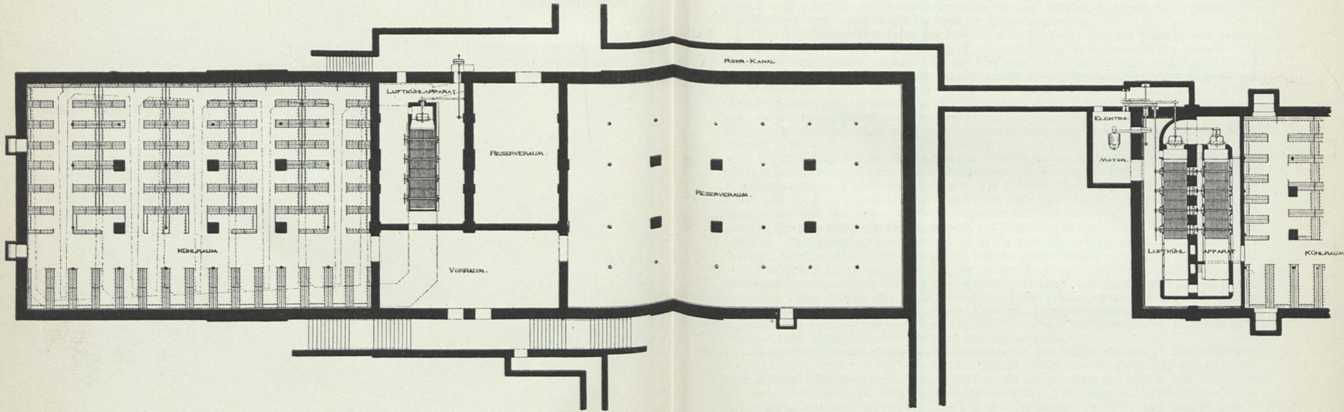
Kühlräume unter der (neuen) Großvieh-Schlachthalle II.
