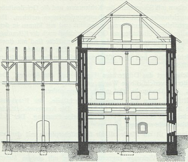
Längenschnitt zu Fig. 140 s1 ).
