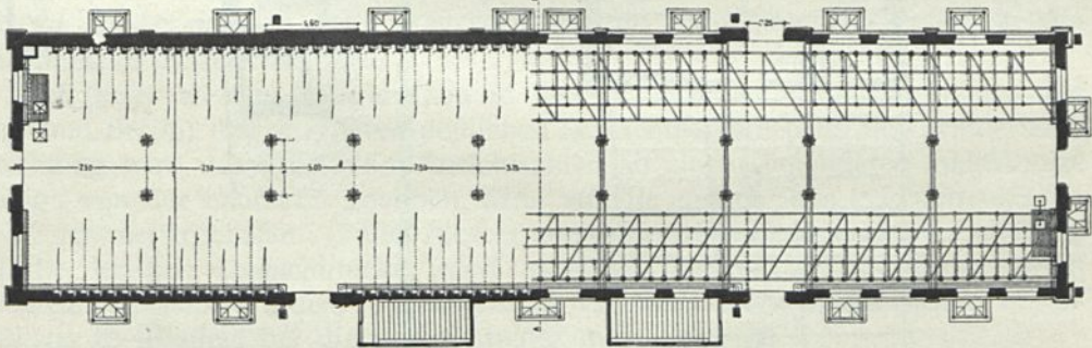
Grundriß der (älteren) Großvieh-Schlachthalle I mit dem darunter gelegenen Kühlräume auf dem Schlachthof zu Nürnberg 30) .
