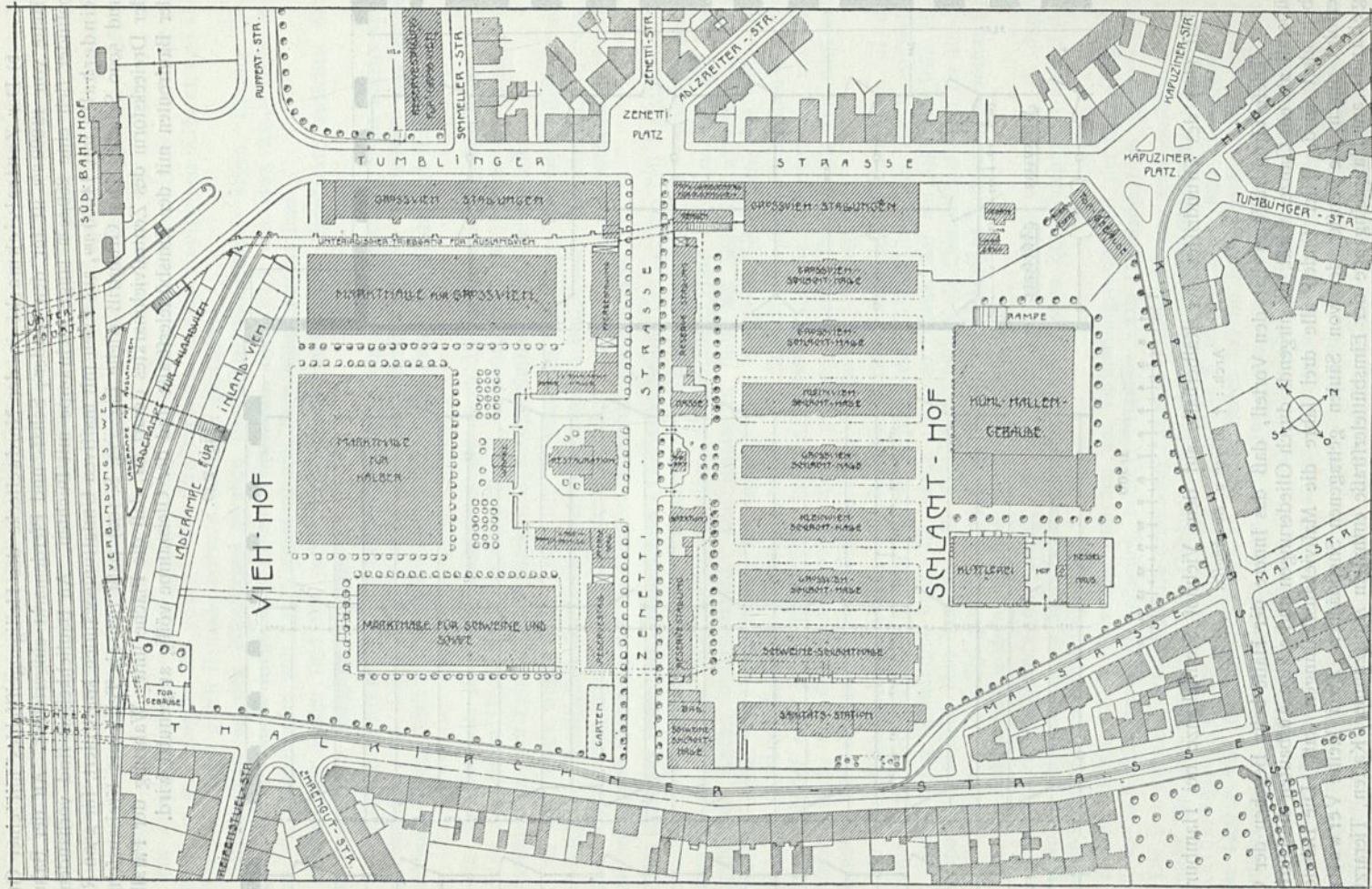
Schlachthof und Viehmarkt zu München 66) .
