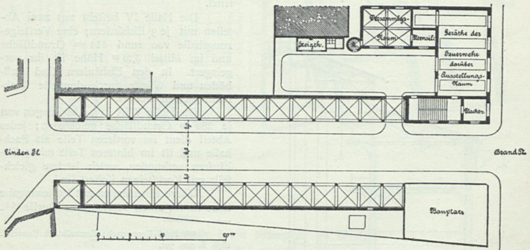
Markthallen und Magazin für Feuerlöfchgeräte zu Gießen 245) .
