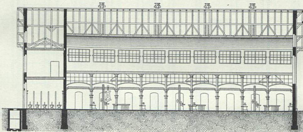
Längsschnitt.
