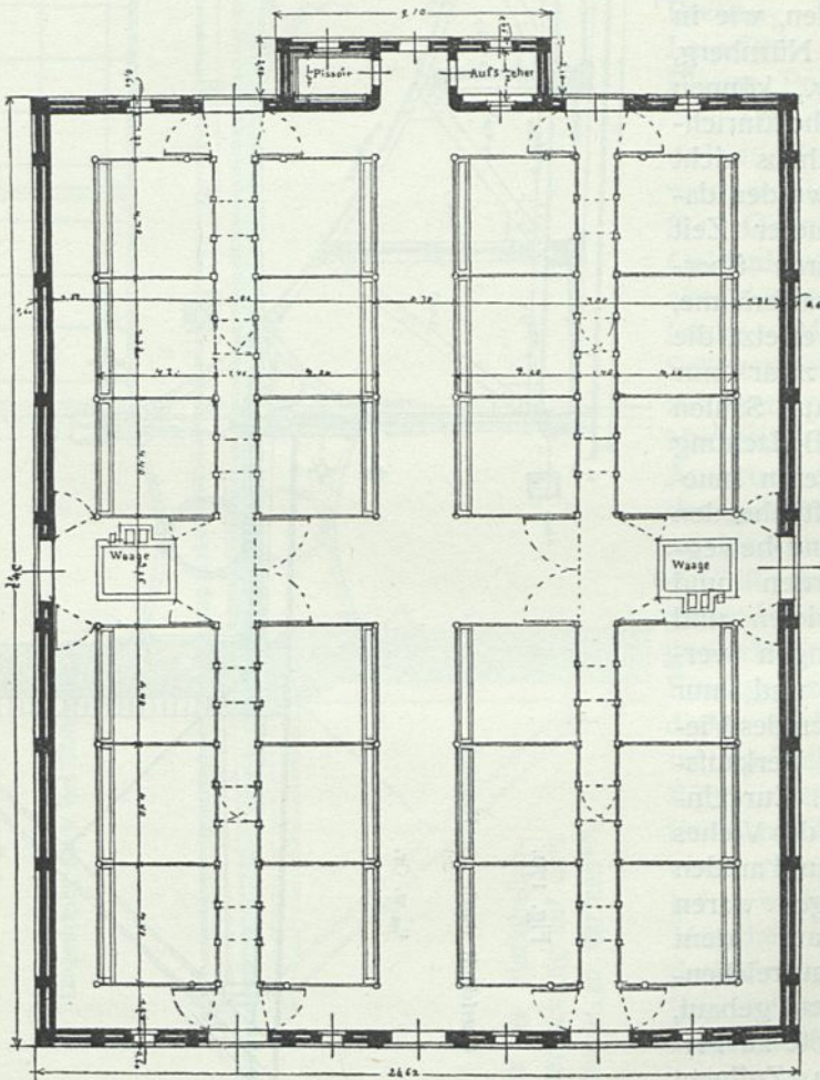
Grundriß.
