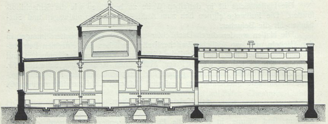
Längenschnitt.
