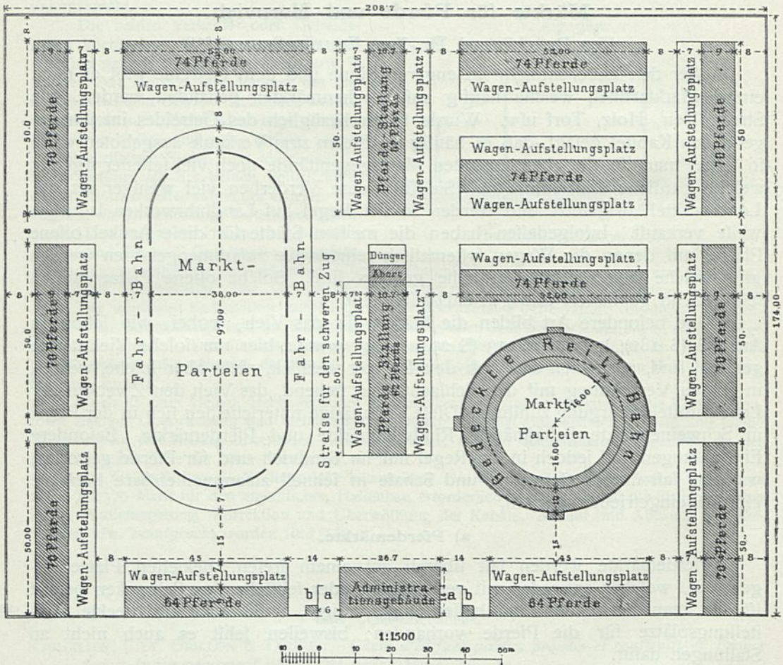
Entwurf für einen Pferdemarkt zu Wien 265) .
