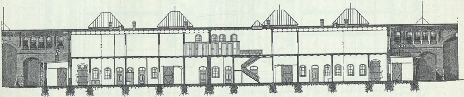
Querchnitt durch die Nebenräume an der Verbindungshalle.
