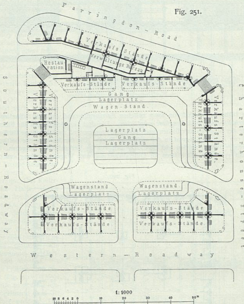
Früchte- und Gemüfemarkt zu London 175) .
