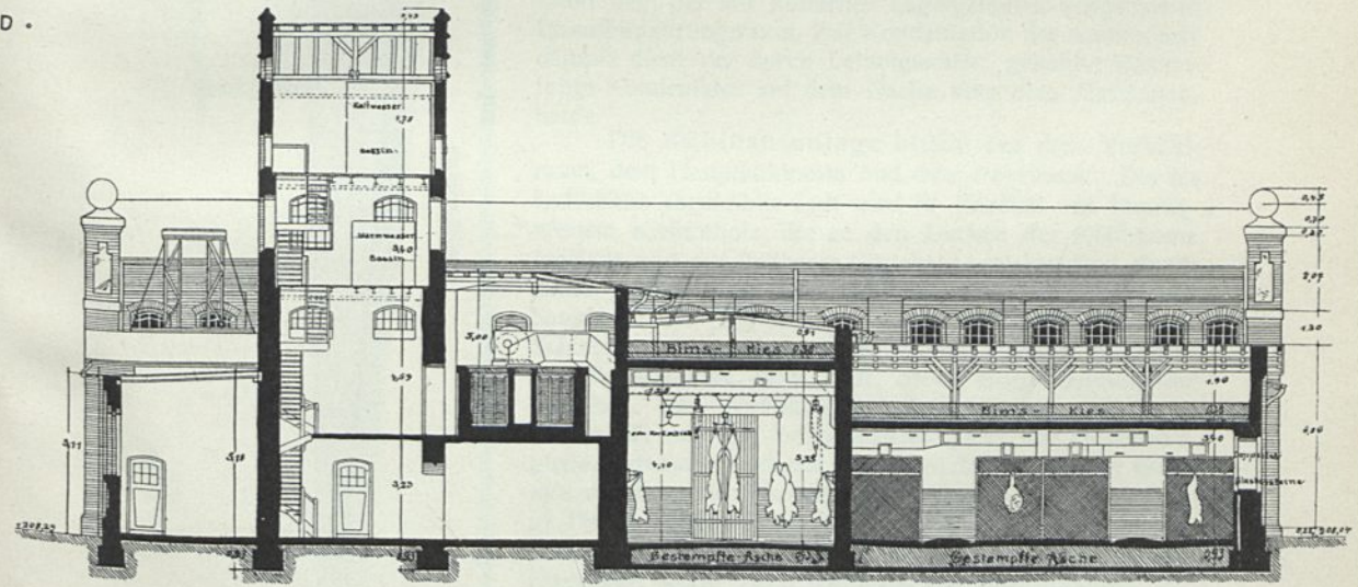
• SCHNITT G-H •
