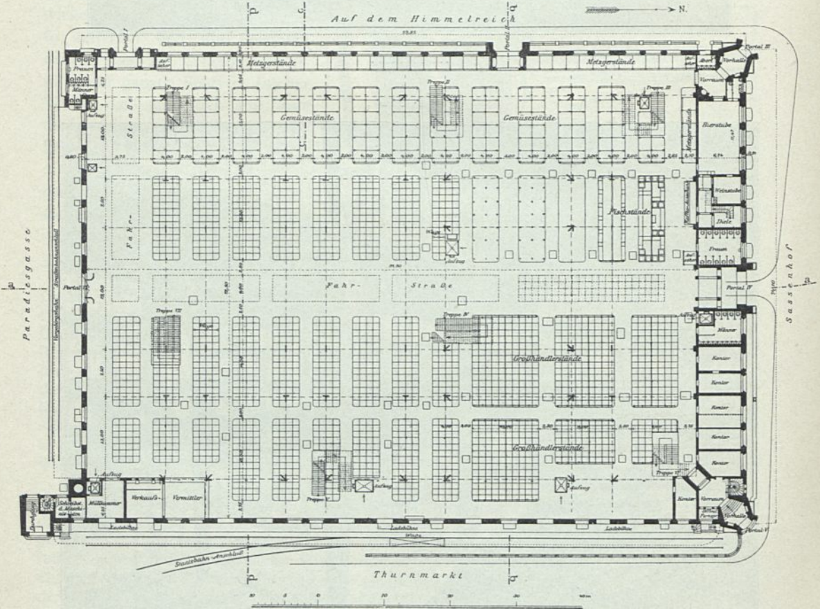
Grundriß.
