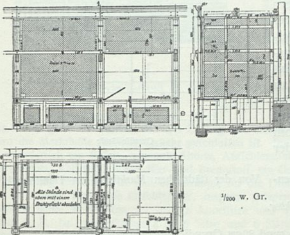
Fleischstand in der städtischen Markthalle zu Hannover 161 ).
