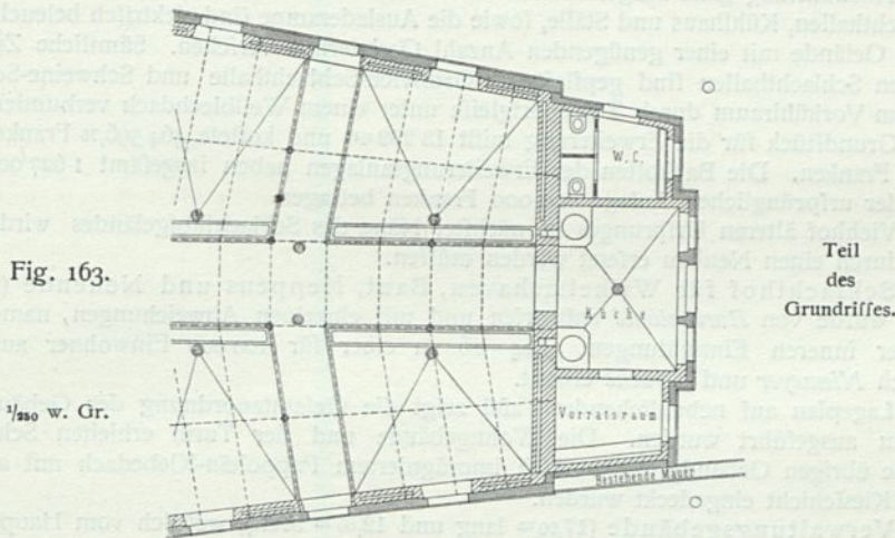
Schweinefall des Schlachthofes zu Basel 90) .
