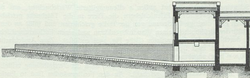
Schnitt durch das Düngerhaus auf dem Schlachthofe zu Schmiedeberg s1 ).
