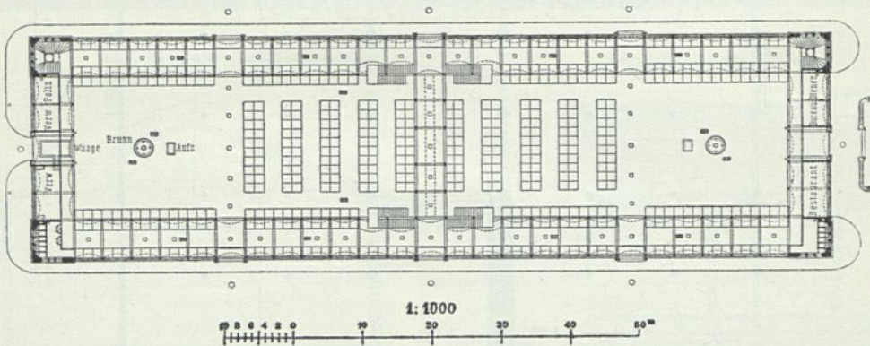
Fig. 366. Kellergeschoß.
