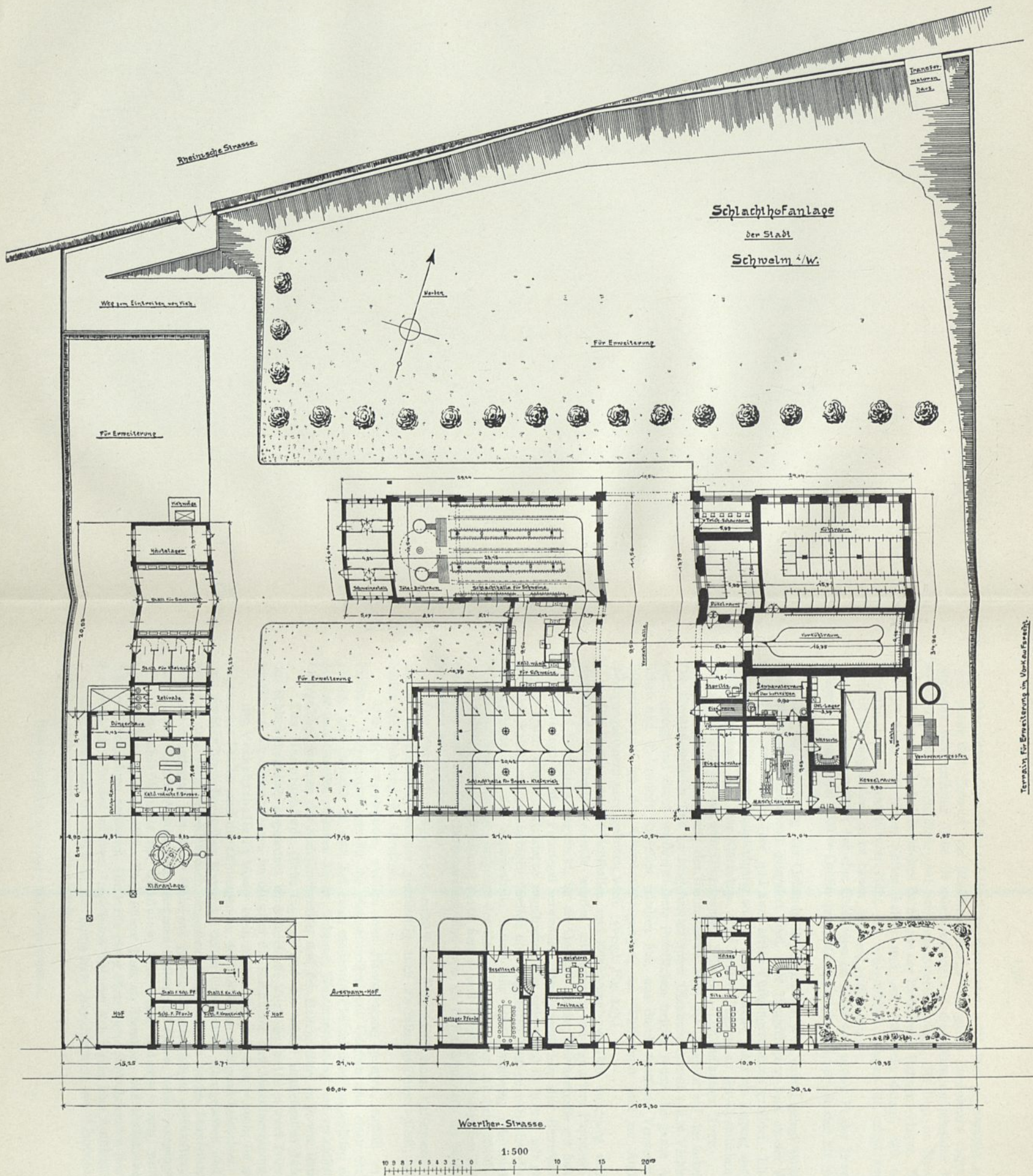
Schlachthof zu Schwelm. Arch.: Bußmann.
