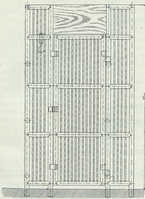
Anficht.
