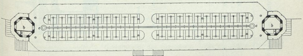
Markthalle für Gemüse, Obst usw. zu Mailand 205 ).
