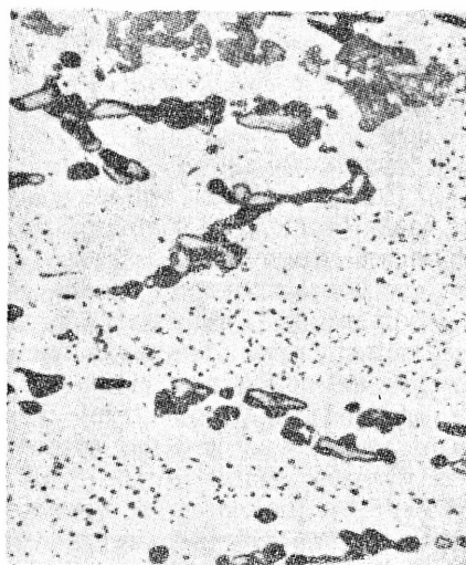
Rys. 4. Mikrostruktura duraluminu, wyciskanego ze zmniejszeniem przekroju 10. Nietraw. \times 500 . Struktura grozdkowa, zupełnie pokruszona.
