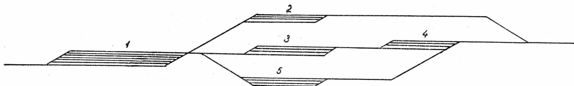
Rys. 2. Schemat bocznic na hucie. Oznaczenia: 1 — hutnicza stacja rozrządcza, 2 — bocznicia koksowni, 3 — bocznicia wielkich pieców, 4 — bocznicia stalowni, 5 — bocznicia walcowni.
