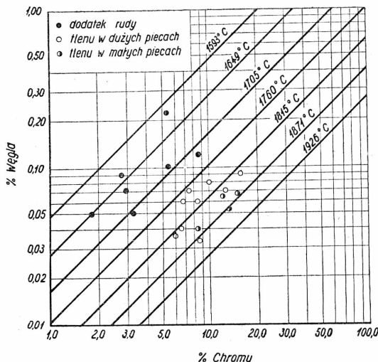
Rys. 3. Temperatury w końcowej fazie świeżenia kąpieli przy dodatku rudy czy też tlenku.
