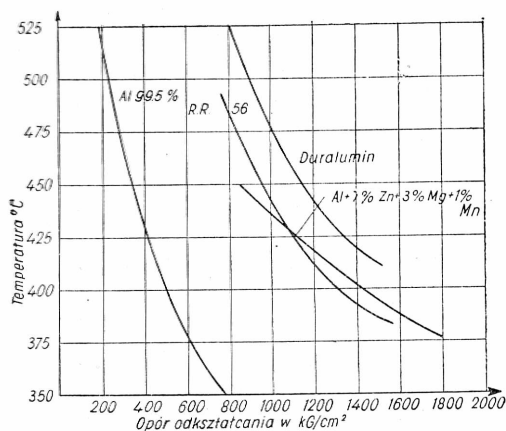
Rys. 1. Opór odkształcania niektórych stopów Al w zależności od temperatury, przy stałej prędkości posuwu tłoka v = 10 cm/min i normalnej matrycy. (C. E. Pearson. Extrusion of Metals, str. 133, Londyn 1944).
