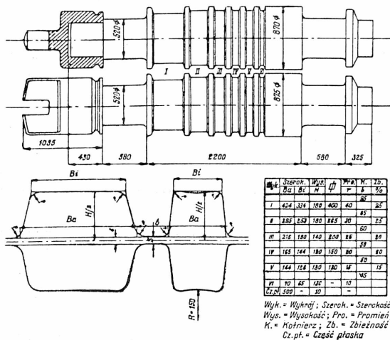
Rys. 4. Walce zgniatacza i ich kalibrowanie.
