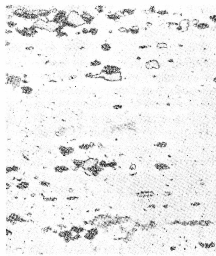
Rys. 3. Mikrostruktura duraluminu, wyciskanego ze zmniejszeniem przekroju 3. Nietraw. \times 500 . Struktura grozdkowa, wydłużona w kierunku wyciskania, ale nie pokruszona.
