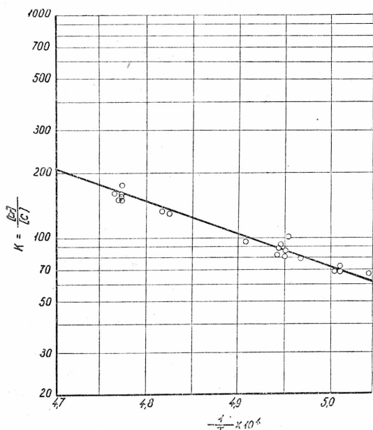
Rys. 2. Wpływ temperatur na stałą równowagi
