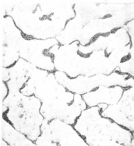
Rys. 2. Mikrostruktura duraluminu, odlanego we wlewnicy. Nietraw. \times 500 .
