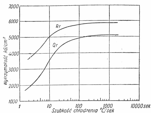
Rys. 8. Wpływ szybkości chłodzenia podczas hartowania na granicę plastyczności i wytrzymałości stopu 75 S. (Cu 1,64%, Mn 0,16%, Mg 2,58%, Zn 5,66%, Cr 0,27%). Stop starzony 24 godz. przy 120° C. (W. L. Fink i L. W. Willey. Metals Technology, sierpień 1947).
