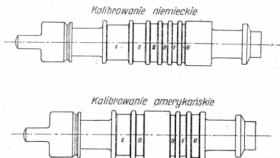
Rys. 3. Walce zgniatacza niemieckiego i amerykańskiego stosowane do walcowania tych samych stali.
