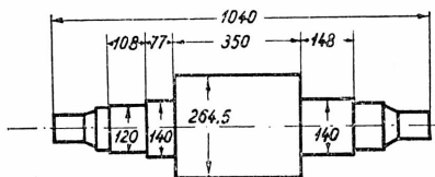
Walec z łożyskami rolkowymi
