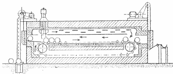
Rys. 6. Piec elektryczny do podgrzewania wlewów, z ruchomym trzonem.
